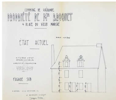
Croquis de la façade sud. Dessin de J. Lucas, 1965. Autr. Jacques Lucas, Phot. Denis (reproduction) Pillet IVR52_20104400659NUCA
