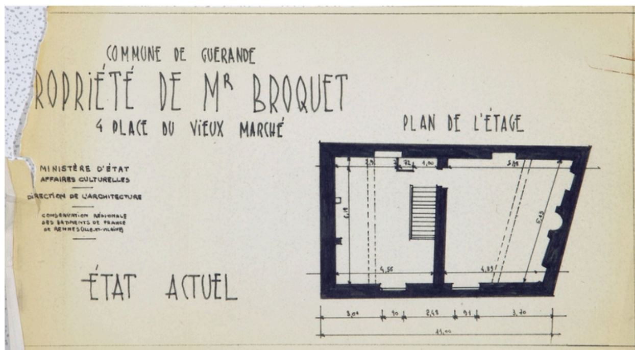
Plan de l'étage. Dessin de J. Lucas, 1965.
