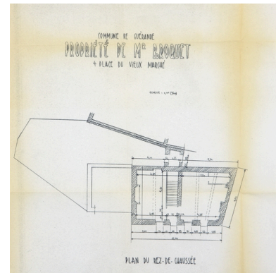
Plan du rez-de-chaussée. Dessin de J. Lucas, 1965. Autr. Jacques Lucas, Phot. Denis (reproduction) Pillet IVR52_20104400660NUCA
