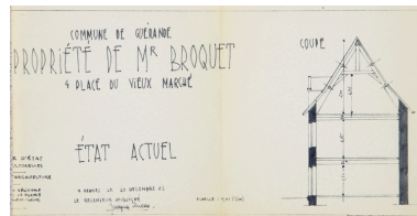
Coupe de la maison. Dessin de J. Lucas, 1965. Autr. Jacques Lucas, Phot. Denis (reproduction) Pillet IVR52_20104400657NUCA
