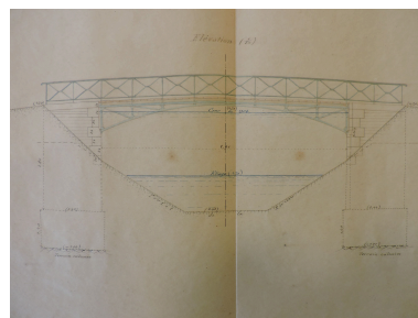
Projet de reconstruction de la passerelle, par le conducteur Texier, 13 février 1905 : élévation. Phot. Yannis (reproduction) Suire IVR52_20218501481NUCA
