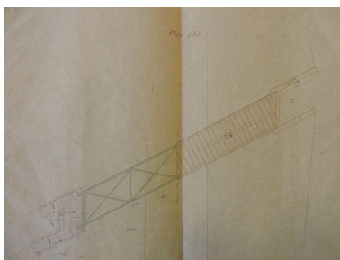
Projet de reconstruction de la passerelle, par le conducteur Texier, 13 février 1905 : plan. Phot. Yannis (reproduction) Suire IVR52_20218501482NUCA
