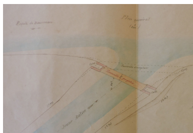
Projet de reconstruction de la passerelle, par le conducteur Texier, 13 février 1905 : plan d'ensemble. Phot. Yannis (reproduction) Suire IVR52_20218501480NUCA
