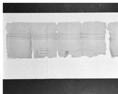
Projet du quai rive gauche, du port de débarquement et du nouveau pont. Elévation du nord (pont neuf) au sud (écluse) et coupes, sixième partie. Autr. Charles Dupuy, Repro. François Lasa IVR52_20025300441X
