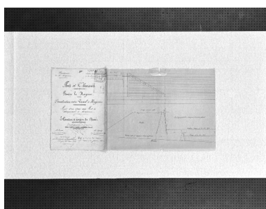
Projet du quai rive gauche, du port de débarquement et du nouveau pont. Elévation du nord (pont neuf) au sud (écluse) et coupes, première partie. Autr. Charles Dupuy, Repro. François Lasa IVR52_20025300446X
