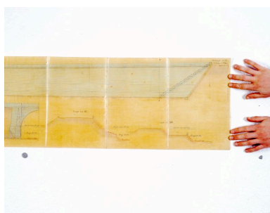
Projet du quai rive droite. Elévation du nord (pont neuf) au sud (écluse) et coupes, sixième partie.
