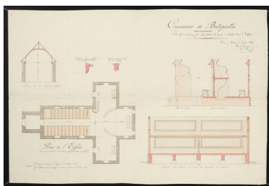
Projet de restauration de l'église de Brétignolles-le-Moulin et dessin des bancs à réaliser, 5 juin 1886. Repro. Morgane Acou-Le Noan IVR52_20205300541NUCA
