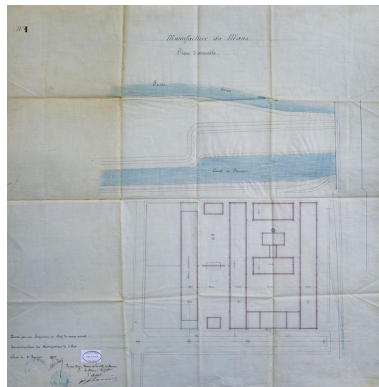
Plan d'assemblage des bâtiments définitifs et provisoires de la manufacture, 1877. Repro. Pierre-Bernard Fourny IVR52_20197202919NUCA
