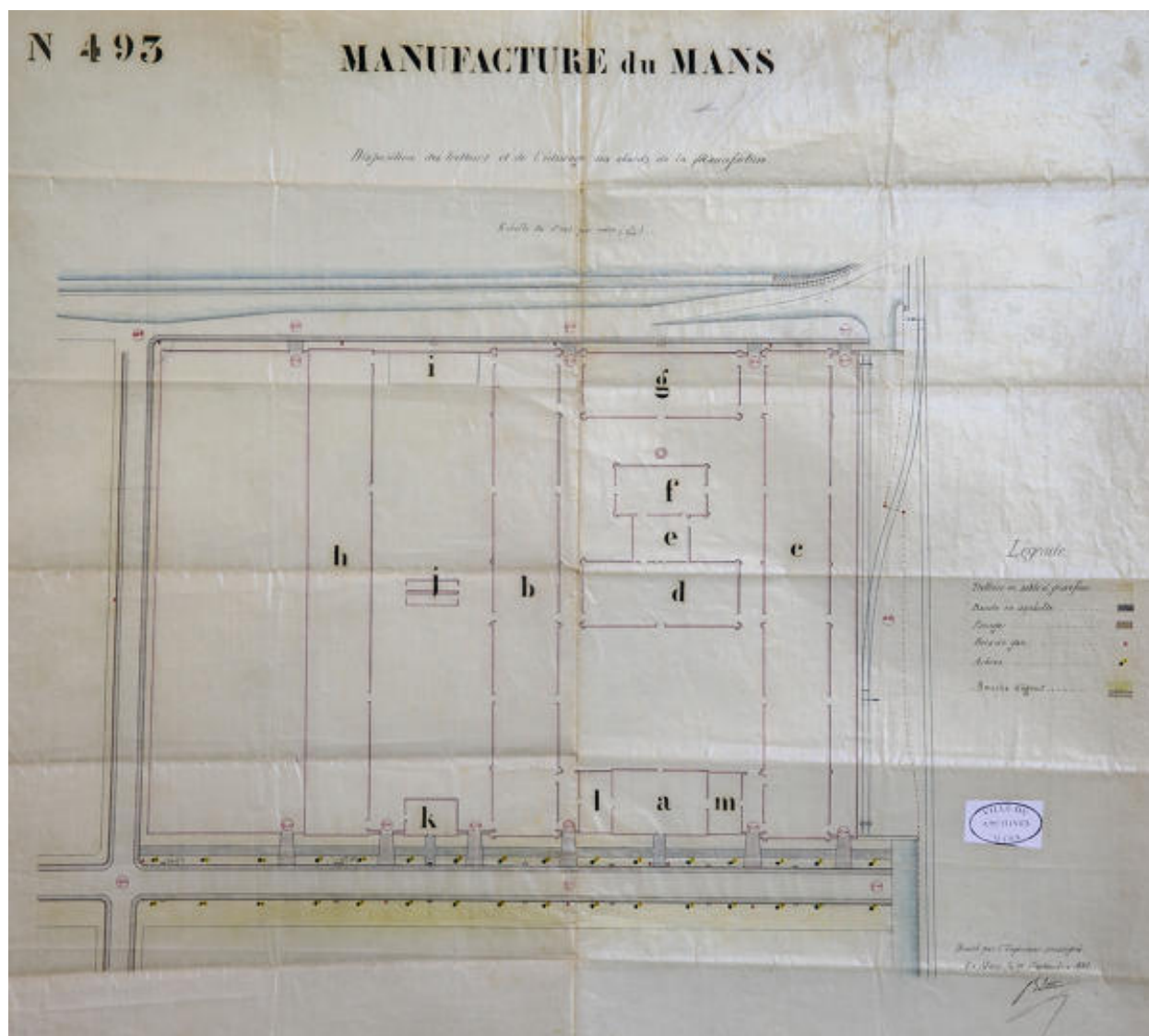
Plan d'aménagement des trottoirs et des éclairages aux abords de la manufacture des Tabacs, 1882.
