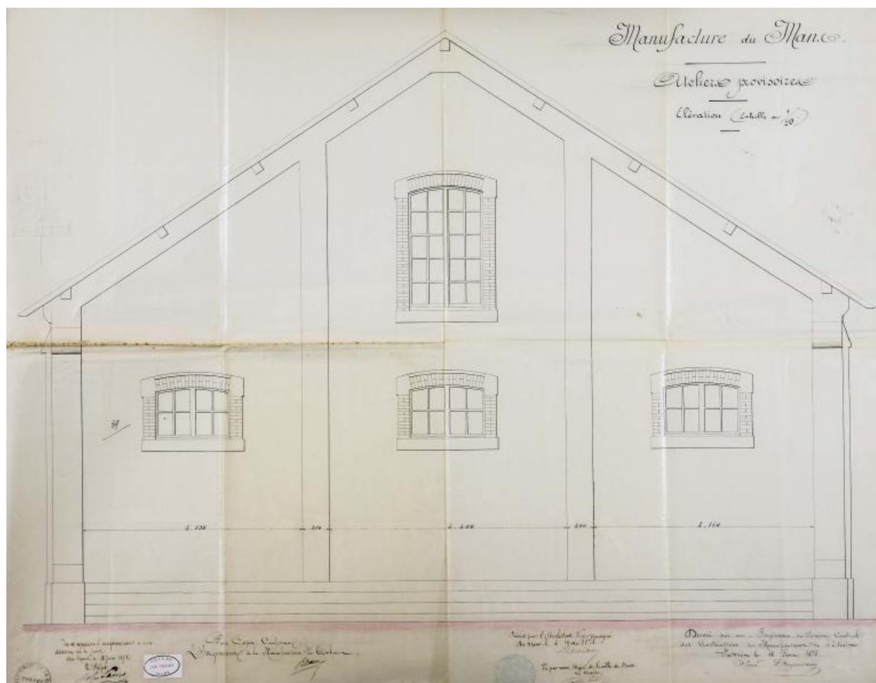
Elévation des ateliers provisoires de la manufacture des tabacs, 1879.
