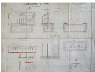
Plan, coupe et élévation pour la construction des lieux d'aisance à la manufacture des Tabacs, 1877. Repro. Pierre-Bernard Fourny IVR52_20197202878NUCA
