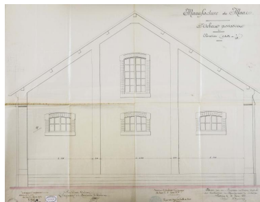
Elévation des ateliers provisoires de la manufacture des tabacs, 1879. Repro. Pierre-Bernard Fourny IVR52_20197200324NUCA
