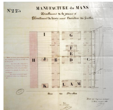
Plan de nivellement des terrains avec positionnement du bâti de la manufacture, 1879. Repro. Pierre-Bernard Fourny IVR52_20197202877NUCA
