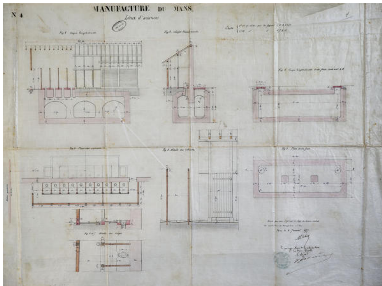
Plan, coupe et élévation pour la construction des lieux d'aisance à la manufacture des Tabacs, 1877.
