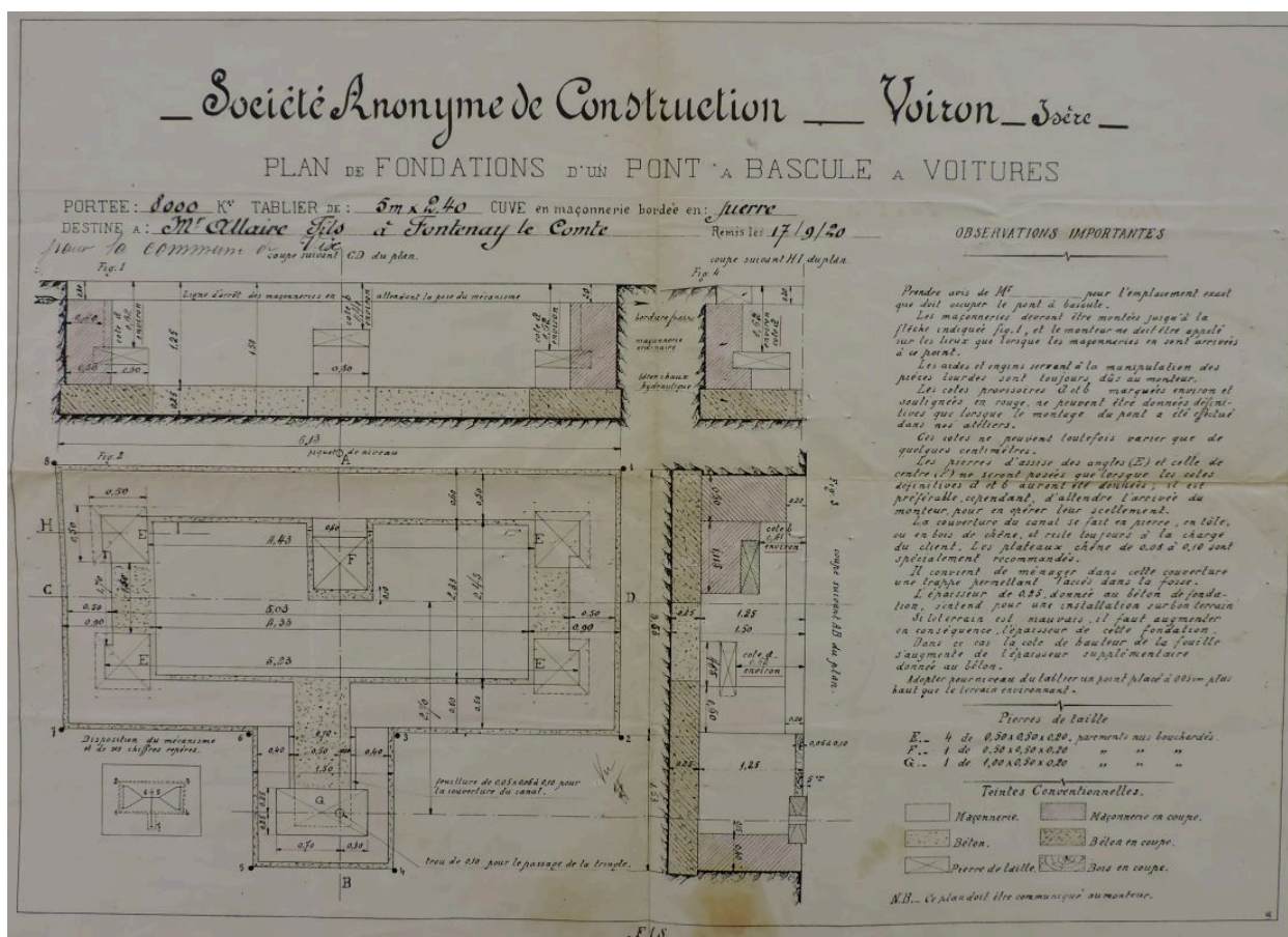
Plan de fondations d'un pont bascule à voitures, par la Société de construction de Voiron, 17 septembre 1920.
