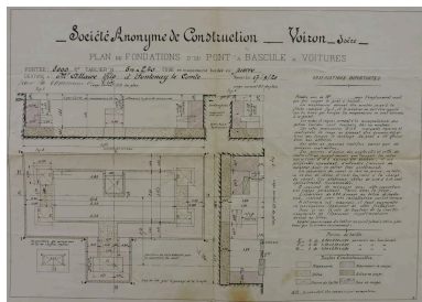
Plan de fondations d'un pont bascule à voitures, par la Société de construction de Voiron, 17 septembre 1920. Phot. Yannis (reproduction) Suire IVR52_20198503631NUCA
