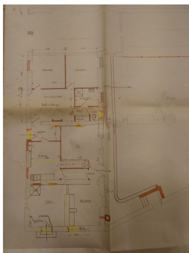
Plan du bureau de poste à l'occasion du réaménagement réalisé en 1960. Phot. Yannis (reproduction) Suire IVR52_20228501097NUCA
