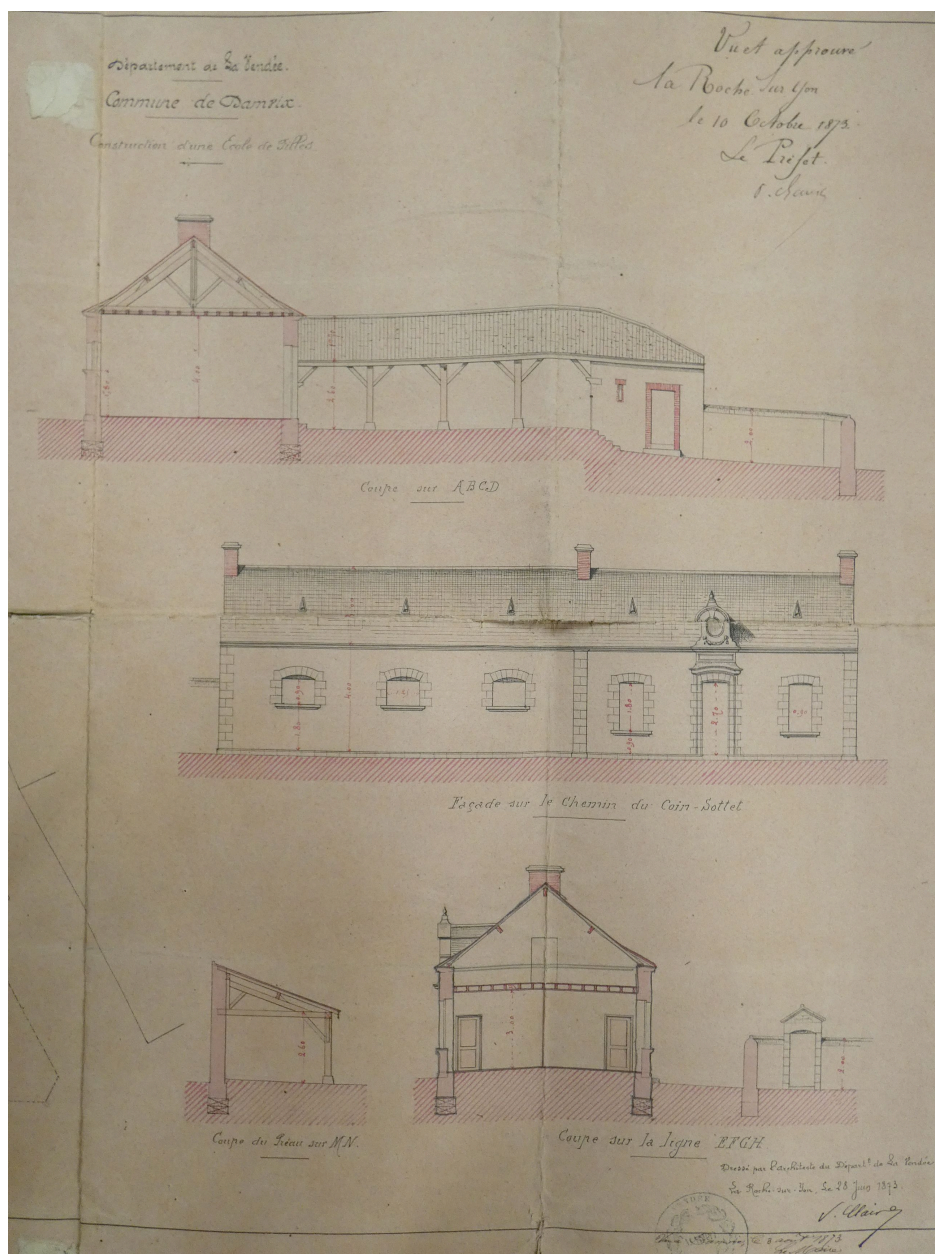
Projet d'école par Victor Clair, 28 juin 1873 : élévations et coupes.
