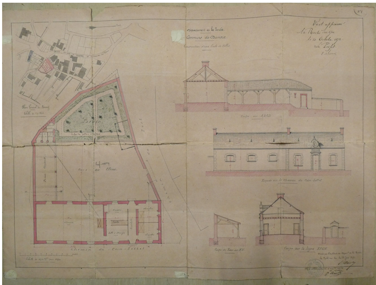
Projet d'école par Victor Clair, 28 juin 1873.
