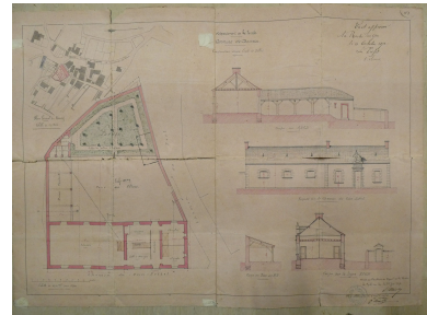
Projet d'école par Victor Clair, 28 juin 1873. Phot. Yannis (reproduction) Suire, Autr. Victor Clair IVR52_20228501121NUCA
