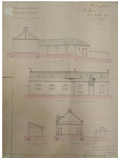
Projet d'école par Victor Clair, 28 juin 1873 : élévations et coupes. Phot. Yannis (reproduction) Suire, Phot. Victor Clair IVR52_20228501123NUCA
