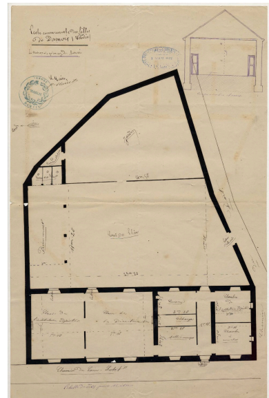
Plan de l'école publique des filles à l'occasion de la création d'un poste d'adjointe, août 1882. Phot. Yannis (reproduction) Suire IVR52_20228501064NUCA
