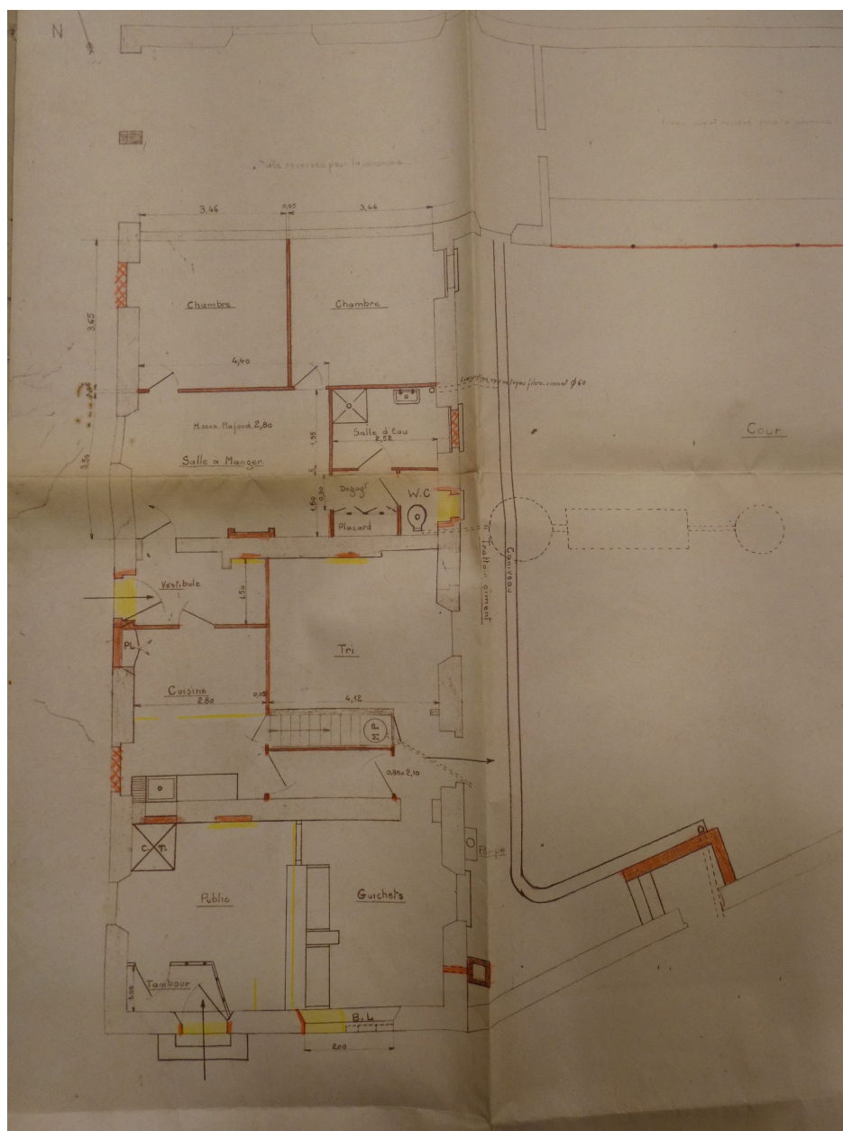
Plan du bureau de poste à l'occasion du réaménagement réalisé en 1960.
