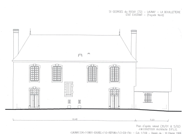
Relevé de l'élévation postérieure du logis en 1999, avant restauration.
