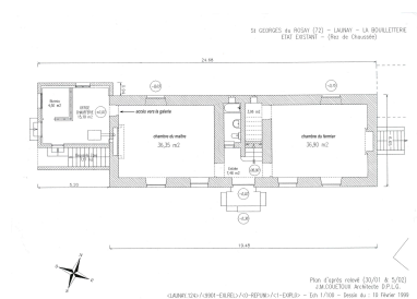
Plan du rez-de-chaussée du logis, avec indication de la distribution d'origine. Dess. Julien Hardy, Autr. J.M. Couetoux IVR52_20157200313NUDAB
