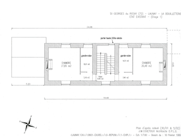
Plan de l'étage du logis, avec indication de la distribution d'origine. Dess. Julien Hardy, Autr. J.M. Couetoux IVR52_20157200314NUDAB
