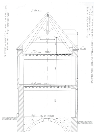
Coupe du logis.
