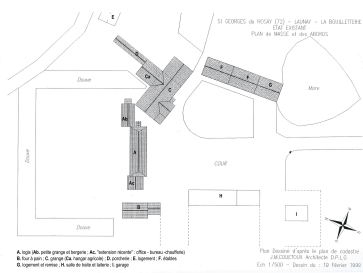
Plan de l'édifice en 1999, avant restauration. A noter les parties agricoles disparues (étables, hangar, laiteries et salles de traite). Dess. Julien Hardy, Autr. J.M. Couetoux IVR52_20157200309NUDAB
