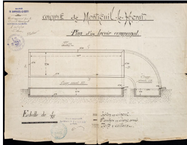
Lavoir communal de Montreuil-le-Henri : plan au sol et coupes, 1921. Repro. Pierre-Bernard Fourny IVR52_20267200027NUCA
