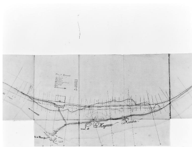
Projet de reconstruction du barrage. Plan d'ensemble : ancienne chaussée (détruite) et barrage projeté, moulin à farine (partiellement reconstruit). Autr. Charles Dupuy, Repro. François Lasa IVR52_20025300178X
