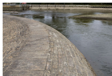
Vue partielle du barrage vers la rive droite, pendant les écourues de 2009.
