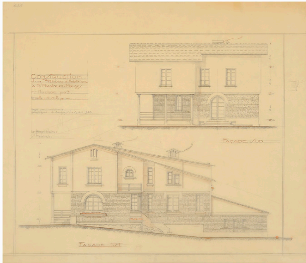
Maison de Louis Huchon : élévations, façade est et sud, par Henry Karcher, architecte, 10 décembre 1948.
