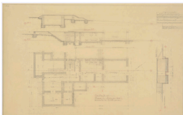
Maison de Louis Huchon : coupe et plan du sous-sol, par Henry Karcher, architecte, 10 décembre 1948. Autr. Henry Karcher IVR52_20114900890NUCA
