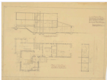
Maison de Louis Huchon : coupe et plan du rez-de- chaussée, par Henry Karcher, architecte, 10 décembre 1948. Autr. Henry Karcher IVR52_20114900891NUCA
