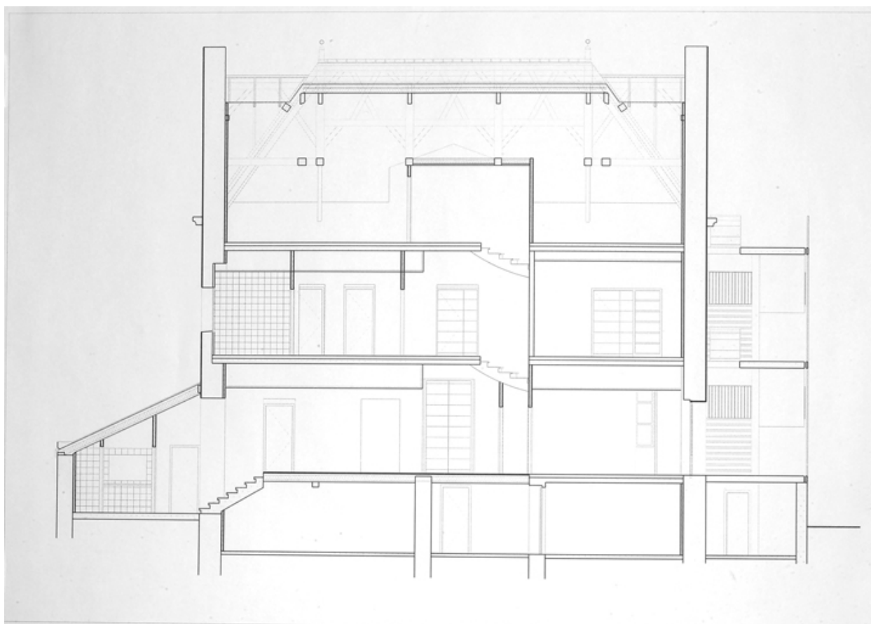
Coupe longitudinale.
