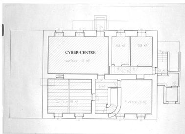
Plan de l'étage de soubassement. Phot. Denis (reproduction) Pillet IVR52_20064401217NUCA
