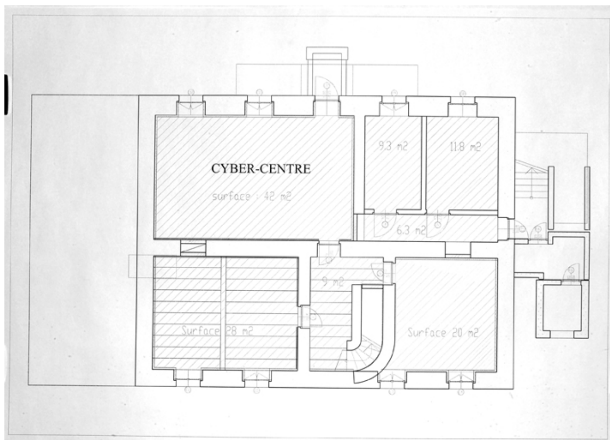
Plan de l'étage de soubassement.
