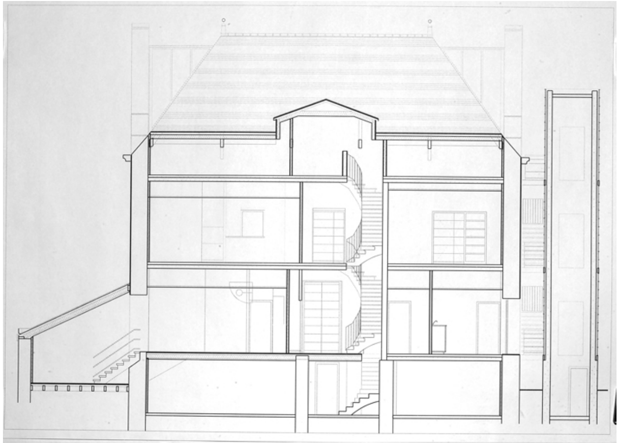
Coupe longitudinale.
