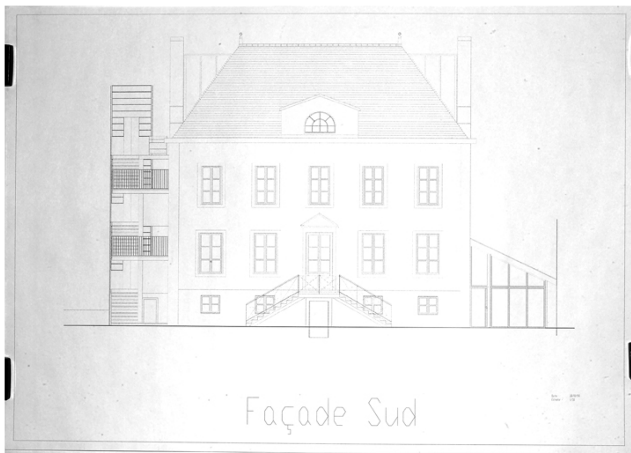
Relevé de la façade sud.
