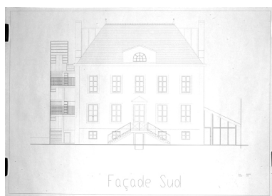
Relevé de la façade sud. Phot. Denis (reproduction) Pillet IVR52_20064401214NUCA
