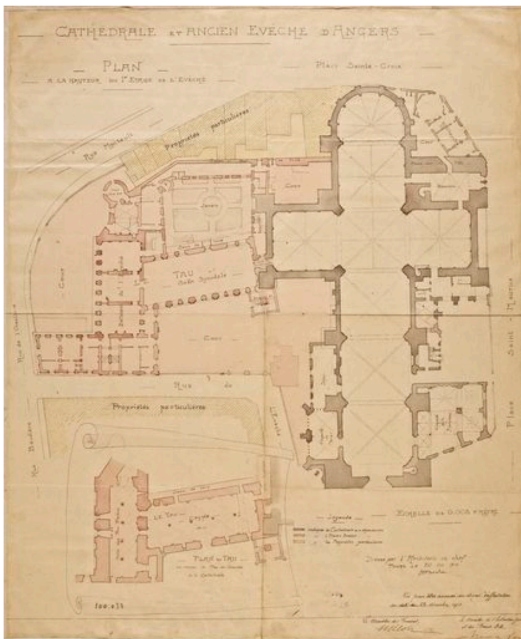
Plan de la cathédrale, plan au 1er étage de l'évêché, plan de la salle basse du Tau, par J. Hardion, 1910.
