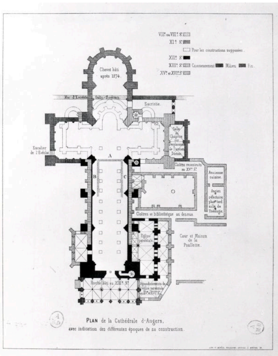
Plan de la cathédrale d'Angers avec indication des différentes époques de construction, lithogr., 1872.
