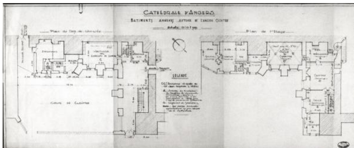
Bâtiments annexes autour de l'ancien cloître : plans du rez-de-chaussée et de l'étage. Dessin, [v. 1950], éch. 1 : 100. 27,5 x 67 cm. (Médiathèque de l'Architecture et du Patrimoine ; 55667).
