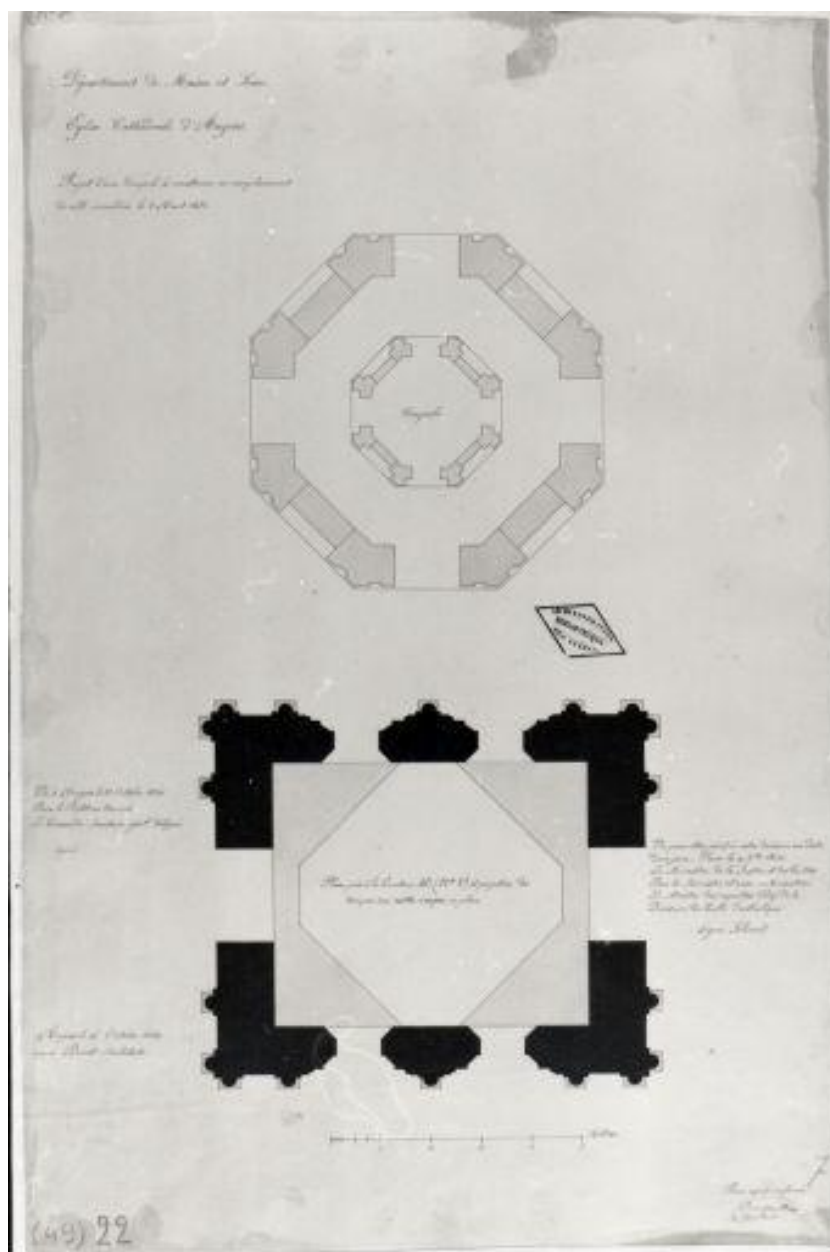
Projet de reconstruction du clocher central : plans de la chambre des cloches et du dôme, par Mathurin Binet, 1836. Dessin, éch. 1 : 50. 49 x 33 cm. (Médiathèque de l'Architecture et du Patrimoine ; 49/2.2).
