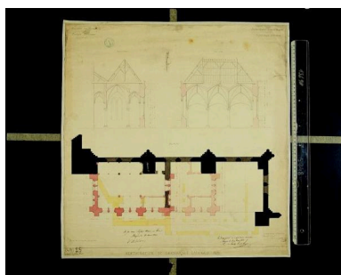
Projet de restauration de la chapelle latérale sud (église paroissiale Saint-Maurice), plan avec indications des parties à détruire et reconstruire, coupes longitudinale et transversale de la nouvelle chapelle, par Charles Joly-Leterme. Dessin, 1852, éch. 1 : 100. 60,5 x 58,5 cm. (Médiathèque de l'Architecture et du Patrimoine ; 49/2.5). Repro. François Lasa IVR52_19934903011X
