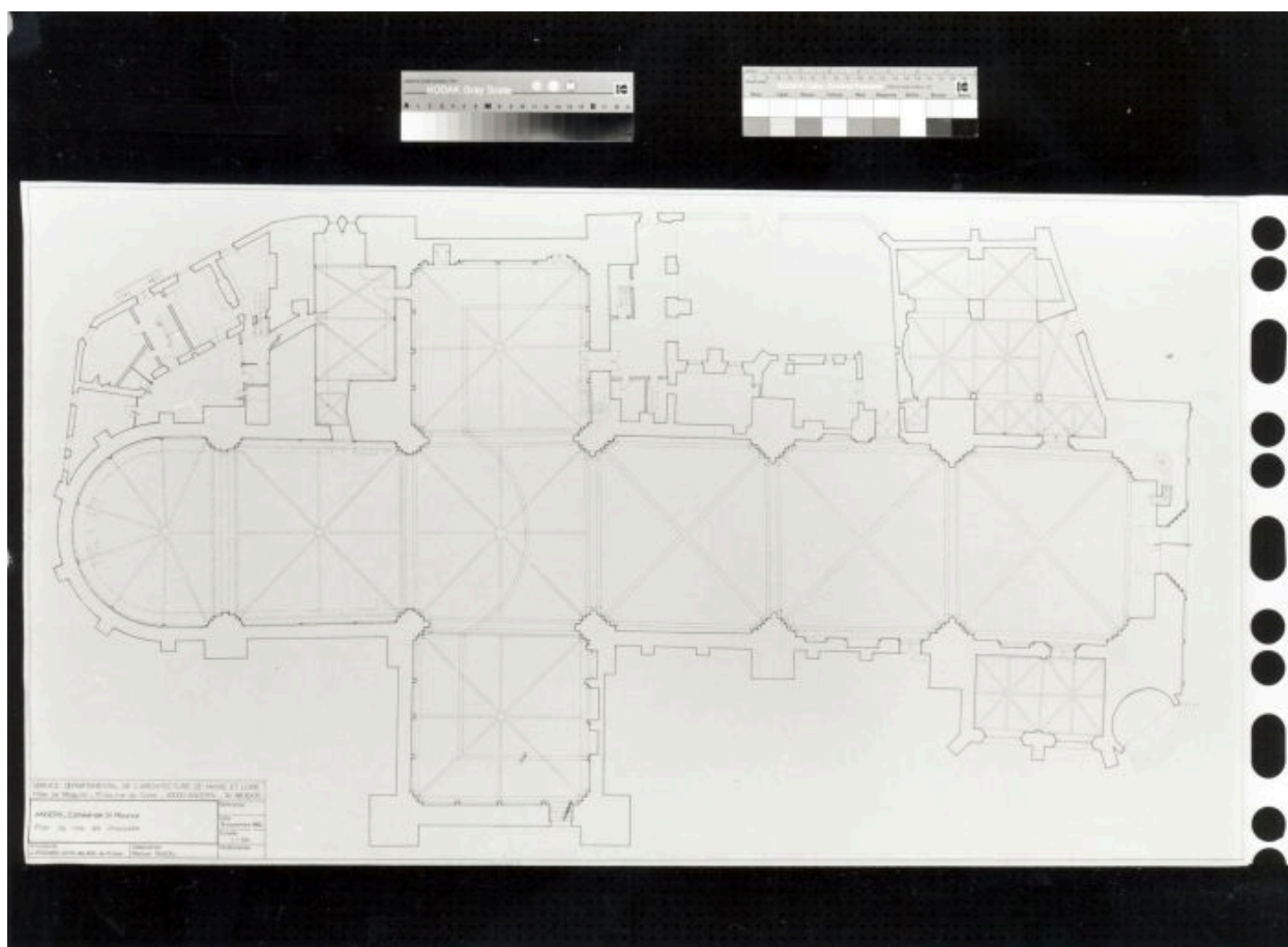
Plan du rez-de-chaussée, par J. Voizard, 1983.
