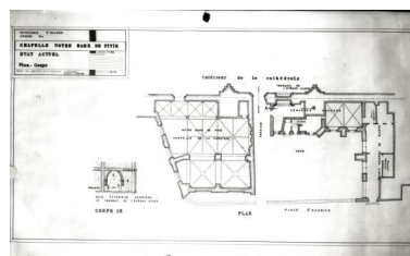
Chapelle Notre-Dame de Pitié [et cloître]. Etat actuel. Plan, coupe, par H. Enguehard. Relevé de plan, 3 fév. 1964, éch. 1 : 100.
