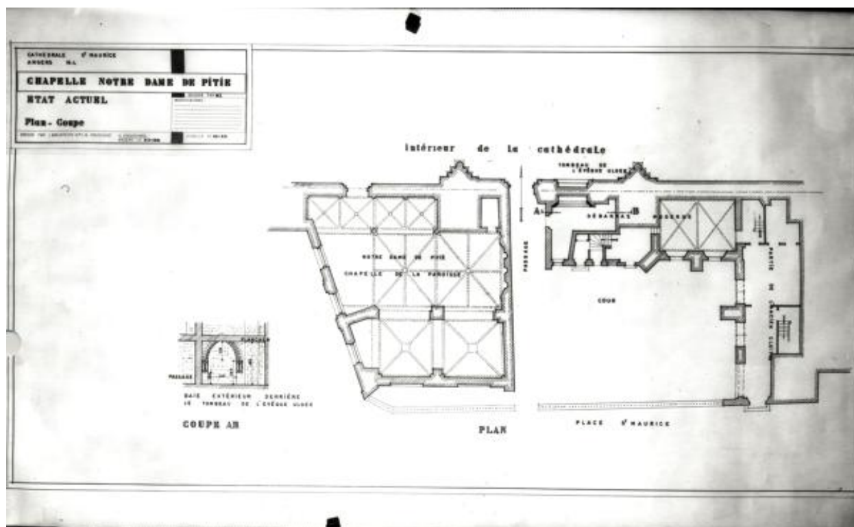
Chapelle Notre-Dame de Pitié [et cloître]. Etat actuel. Plan, coupe, par H. Enguehard. Relevé de plan, 3 fév. 1964, éch. 1 : 100.
