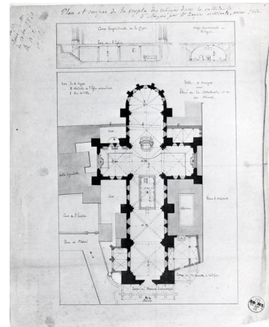
Plan et coupes de la crypte des Evêques dans la cathédrale d'Angers, par Ch.-Paul Rocques, 1860. Repro. François Lasa, Autr. Charles-Paul Rocques IVR52_19794900545X
