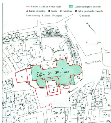
Plan-masse et de situation. D'après le plan cadastral, 1840, section J, parcelle 369, éch. 1 : 1 000. Dess. I. Frager IVR52_20034900971A4
