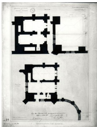
Projet de sacristie et de salle capitulaire : plans du soubassement, du rez-de-chaussée et des couvertures, par Charles Joly-Leterme, 1852. Dessin, éch. 1 : 100. 65 x 49,5 cm. (Médiathèque de l'Architecture et du Patrimoine ; 4929). Repro. François Lasa IVR52_19934903023X
