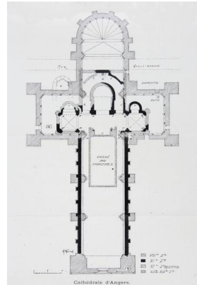
Plan des fouilles de 1902. Repro. François Lasa IVR52_20064902957NUCA
