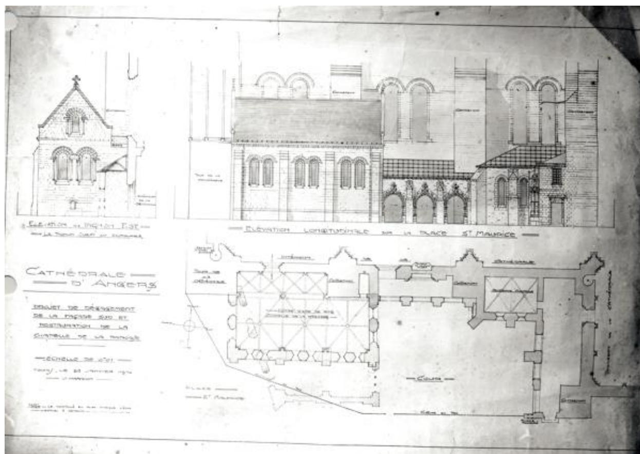
Projet de dégagement de la façade sud et restauration de la chapelle de la paroisse : plan et élévations par Jean Hardion. Dessin, 25 janv. 1914. (Collection particulière, Henri Enguehard).
