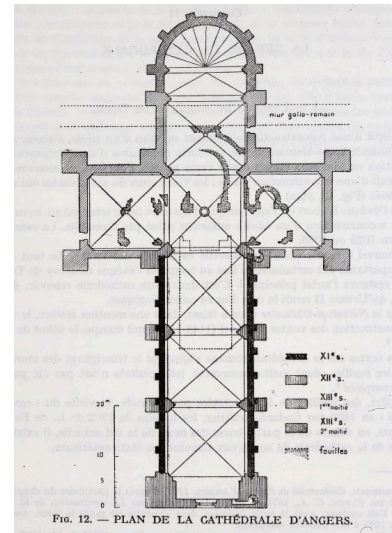
Plan de la cathédrale, avec ses différentes campagnes de construction, vers 1963. Repro. François Lasa IVR52_20064902898NUCA
