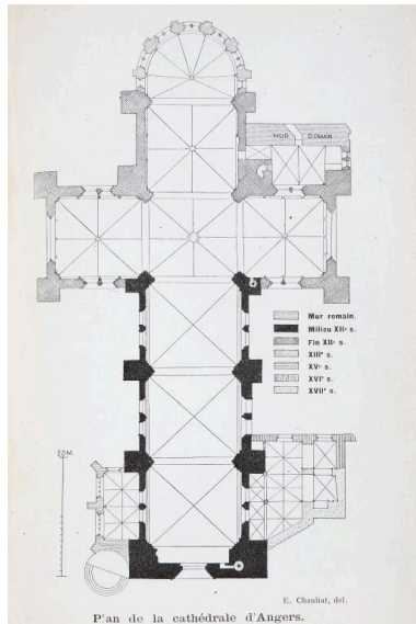
Plan de la cathédrale d'Angers, par E. Chauliat, 1910. Autr. E. Chauliat, Repro. François Lasa IVR52_20064902956NUCA
