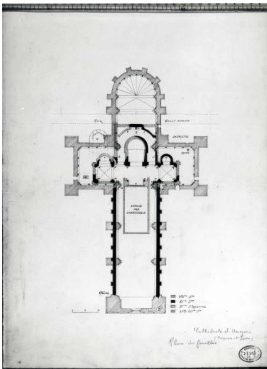
Cathédrale d'Angers (Maine-et-Loire). Plan des fouilles [de 1902].
