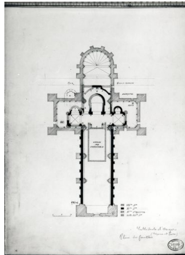
Cathédrale d'Angers (Maine-et-Loire). Plan des fouilles [de 1902]. Repro. François Lasa IVR52_19934902995X
