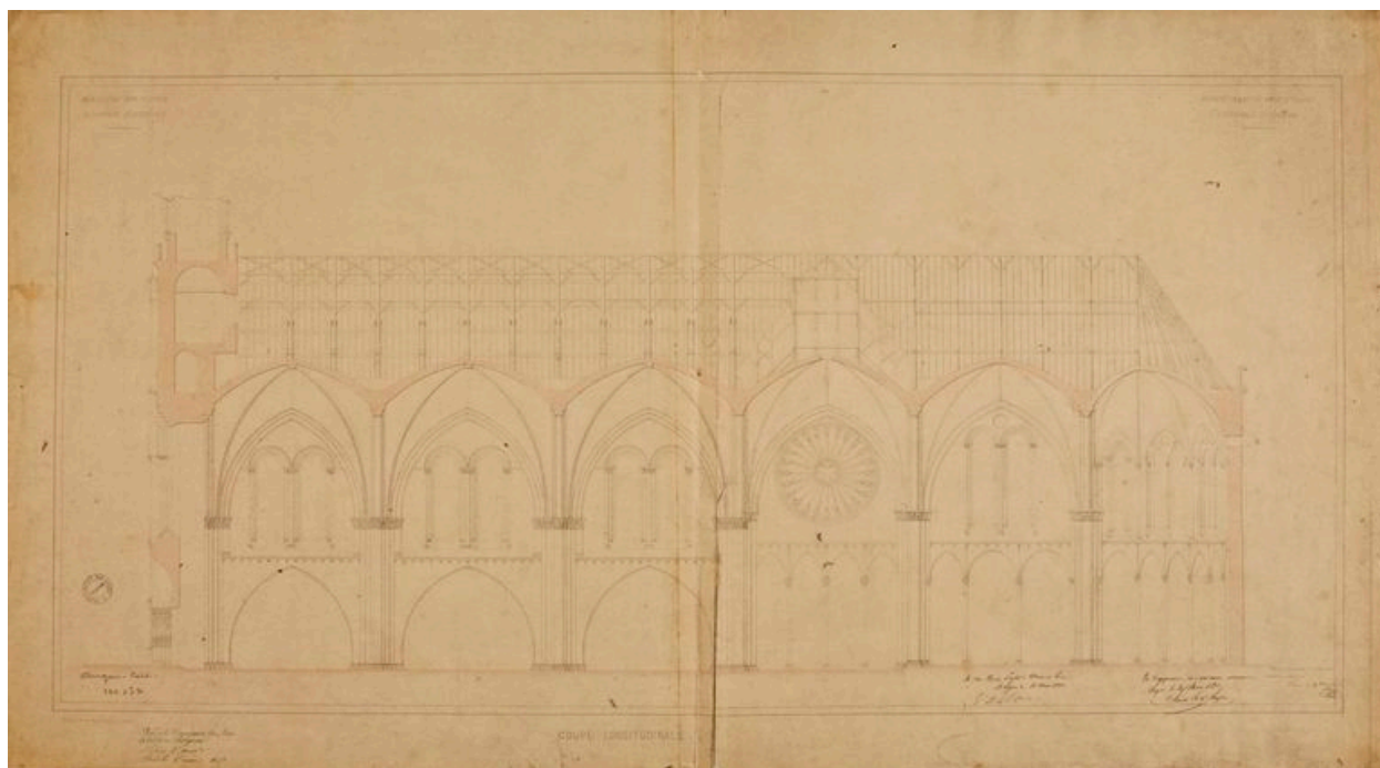
Coupe longitudinale, par Ch. Joly-Leterme, 1852.
