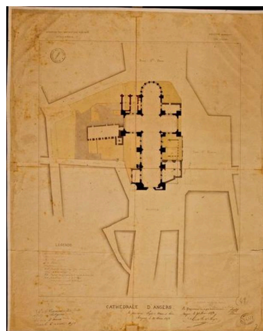
Plan de la cathédrale, avec les parties du cloître à détruire et les constructions neuves en projet (sacristie et salle capitulaire au nord-est, chapelle latérale au sud- ouest), par Ch. Joly-Leterme, 1849. Repro. François Lasa, Autr. Charles Joly-Leterme IVR52_19934903026XA
