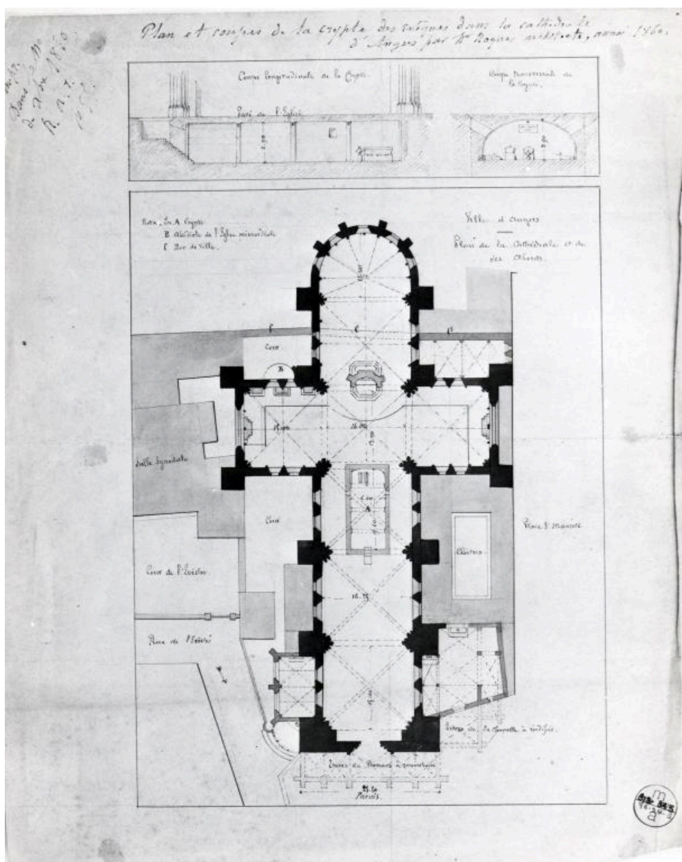
Plan et coupes de la crypte des Evêques dans la cathédrale d'Angers, par Ch.-Paul Rocques, 1860.
