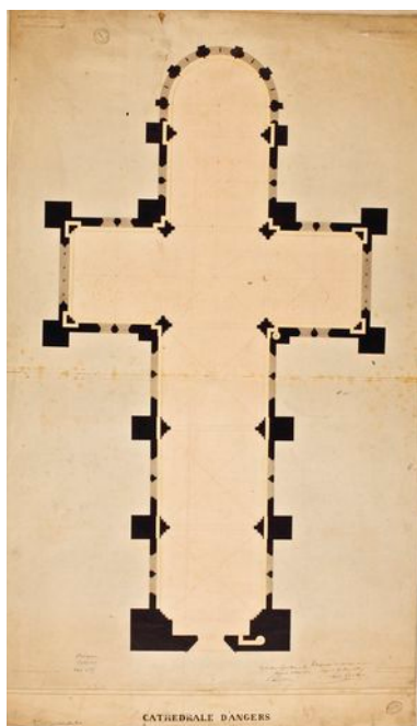
Plan général au-dessus des tribunes, dessin, par Ch. Joly-Leterme, 1852. Repro. François Lasa, Autr. Charles Joly-Leterme IVR52_19934903014XA
