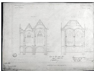
Construction d'une sacristie et d'une salle capitulaire : coupes transversale et longitudinale, par Charles Joly-Leterme, 1853. Dessin, éch. 1 : 100. 44,5 x 60 cm. (Médiathèque de l'Architecture et du Patrimoine ; 49/2.7). Repro. François Lasa IVR52_19934902997X
