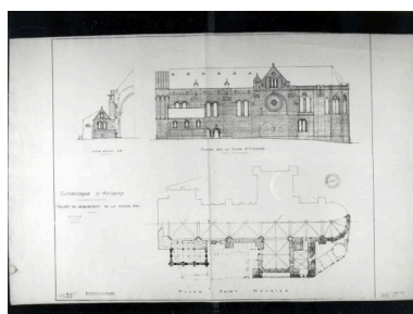
Projet de dégagement de la façade sud : plan et élévations, par A.-M. Pélissier. Dessin, [début 20e siècle], éch. 1 : 200. 65,5 x 101,5 cm. (Médiathèque de l'Architecture et du Patrimoine ; 49/3.51). Repro. François Lasa IVR52_19934903016X
