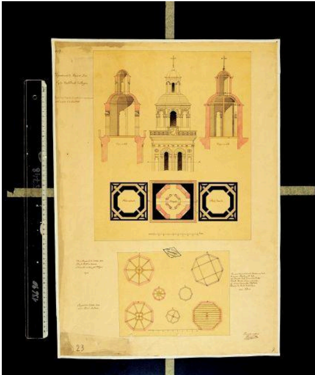
Projet de reconstruction de la partie haute du clocher central, (après incendie de 1831) : plan, coupes et élévation du dôme, par Mathurin Binet, 1836. Dessin, éch. 1 : 100. 66,5 x 46 cm. (Médiathèque de l'Architecture et du Patrimoine ; 49/2.3).
