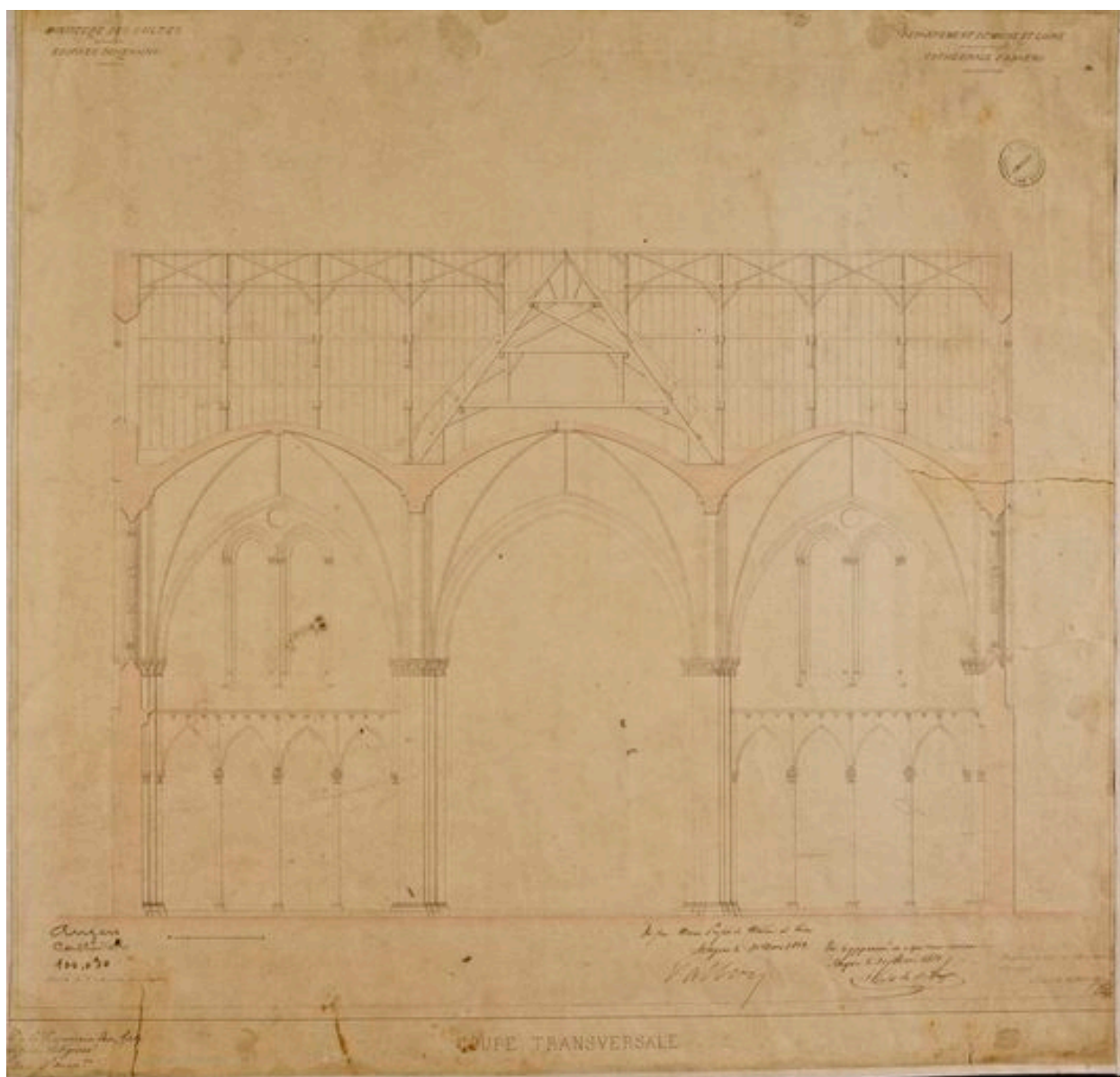
Coupe transversale à la croisée du transept, vers l'est, par Ch. Joly-Leterme, 1852.
