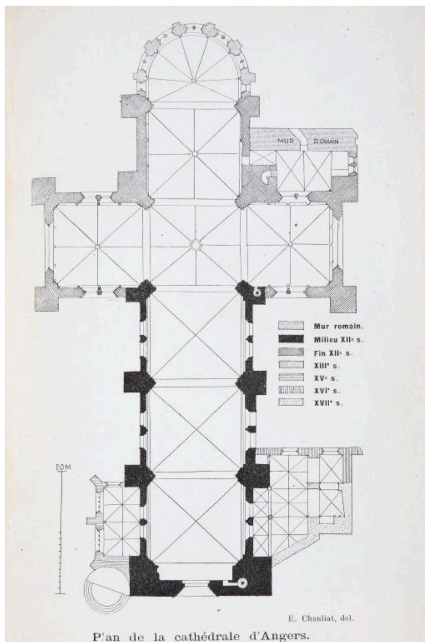
Plan de la cathédrale d'Angers, par E. Chauliat, 1910.
