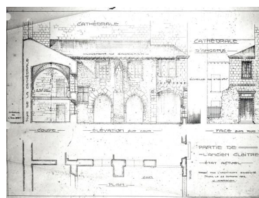
Partie de l'ancien cloître. Etat actuel : aile est, avec coupe sur l'aile nord, par Jean Hardion, 1973. (Collection particulière, Henri Enguehard). Repro. François Lasa IVR52_19754900534P
