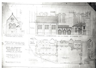
Projet de dégagement de la façade sud et restauration de la chapelle de la paroisse : plan
