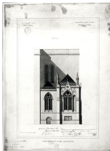
Projet de sacristie et de salle capitulaire : élévation est, par Charles Joly-Leterme, 1852, Dessin, éch. 1 : 100. 58,5 x 42,5 cm.. (Médiathèque de l'Architecture et du Patrimoine). Repro. François Lasa IVR52_19934903024X
