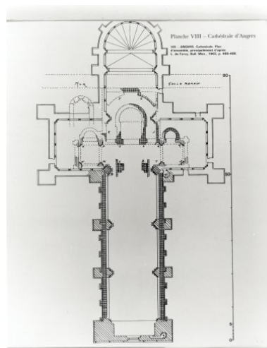
Plan d'ensemble, principalement d'après Louis de Farcy, 1902. Repro. François Lasa IVR52_19954900984X
