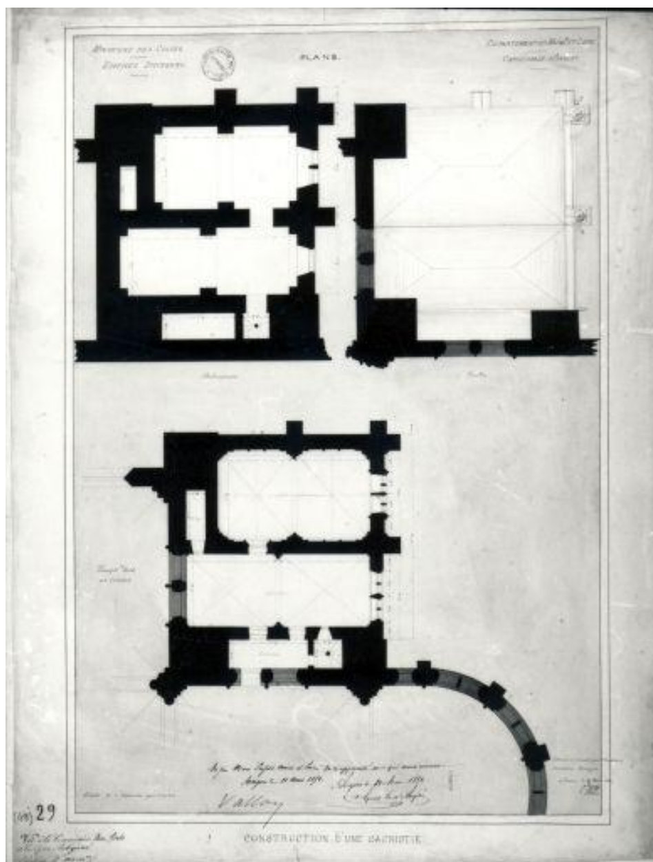
Projet de sacristie et de salle capitulaire : plans du soubassement, du rez-de-chaussée et des couvertures, par Charles Joly-Leterme, 1852. Dessin, éch. 1 : 100. 65 x 49,5 cm. (Médiathèque de l'Architecture et du Patrimoine ; 4929).
