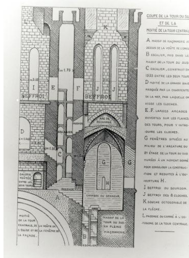
Coupe de la tour du sud et de la moitié de la tour centrale, par L. de Farcy. Relevé imprimé, [début 20e siècle]. In : FARCY, Louis de : "Monographie de la cathédrale d'Angers", Angers : Josselin, A. Bruel, Paris, Bruges : Desclée, De Brouwer, 1910, vol. 1. Repro. François Lasa IVR52_19954900971X
