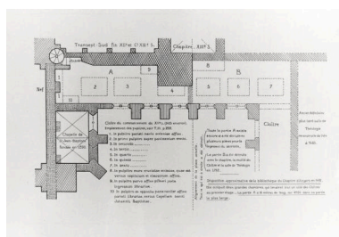
Plan du cloître avec les parties existantes (en A) et détruites en 1792 (en B), par L.ouis de Farcy. Relevé imprimé. In : FARCY, Louis de : "Monographie de la cathédrale d'Angers", Angers : Josselin, A. Bruel, Paris, Bruges : Impr. de Brouwer, 1910, vol. 1. Repro. François Lasa IVR52_19954900973X
