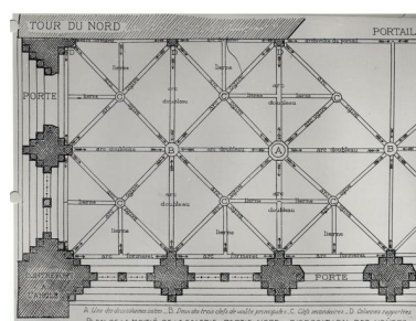
Porche occidental, plan de reconstitution de la partie nord avec le dessin des voûtes, par Louis de Farcy. Dessin à la plume, imprimé, [v. 1910]. 21 x 25,5 cm. In : FARCY, Louis de : "Monographie de la cathédrale d'Angers", Angers : Josselin, A. Bruel, Paris, Bruges : Impr. de Brouwer, 1910, vol. 1. Repro. François Lasa IVR52_19984902563X
