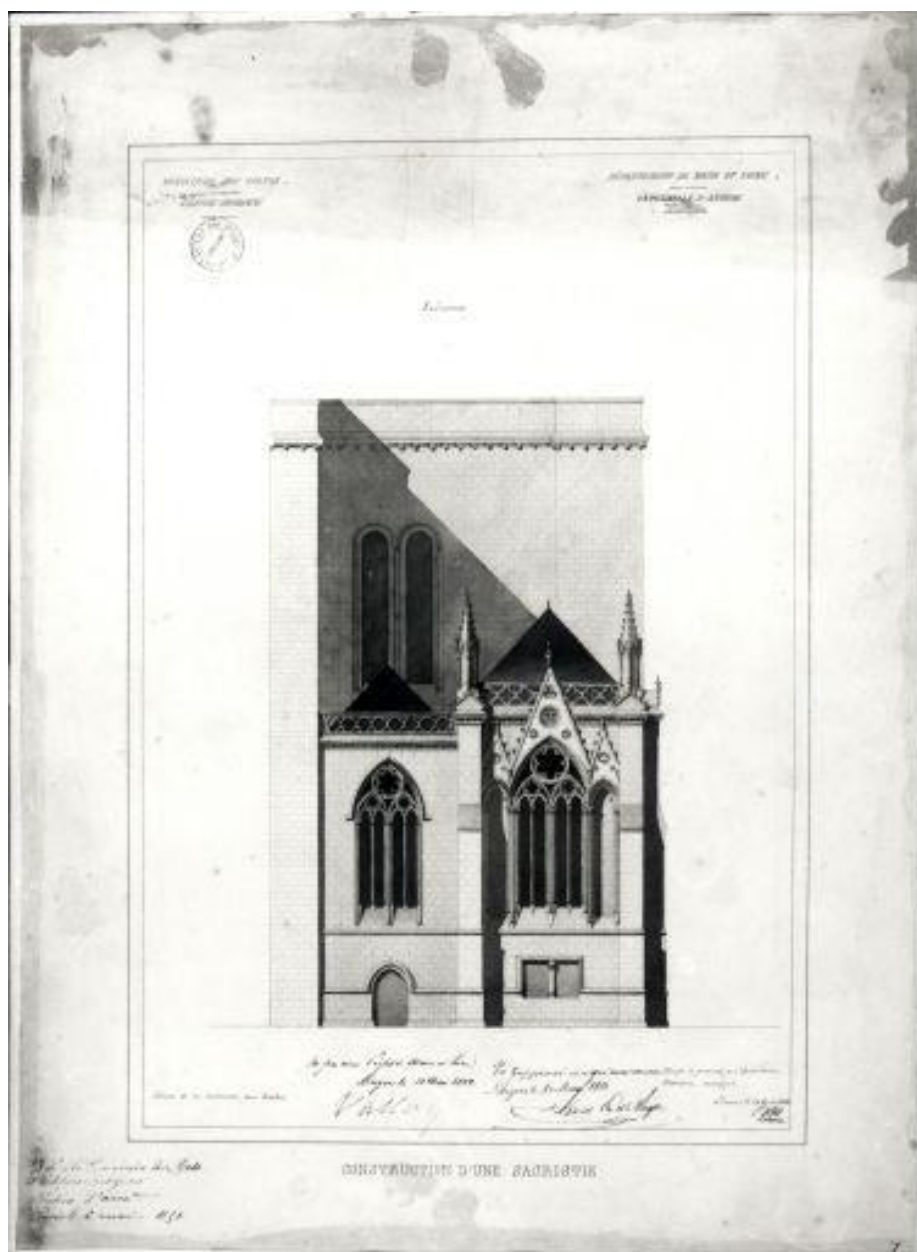
Projet de sacristie et de salle capitulaire : élévation est, par Charles Joly-Leterme, 1852, Dessin, éch. 1 : 100. 58,5 x 42,5 cm.. (Médiathèque de l'Architecture et du Patrimoine).
