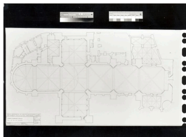
Plan du rez-de-chaussée, par J. Voizard, 1983. Repro. François Lasa, Autr. Jean Voizard IVR52_19954900813X
