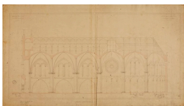
Coupe longitudinale, par Ch. Joly-Leterme, 1852. Repro. François Lasa, Autr. Charles Joly-Leterme IVR52_19934903015XA
