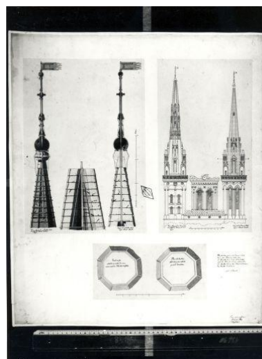
Restauration de la flèche sud : plan, coupe, élévation. Elévation des flèches et du clocher central après l'incendie de 1831, dessin, éch. 0,014 pm, 0,051 pm, 0,007 pm. par Mathurin Binet, 1836. (Médiathèque de l'Architecture et du Patrimoine). Repro. François Lasa IVR52_19934903008X
