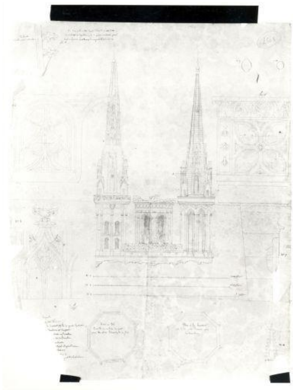
Restauration des flèches : plan et élévation, par l'architecte Louis François [dit François Père], [v. 1829]. Dessin, 54,2 x 42 cm. (AD Maine-et-Loire ; 90 J 2508).
