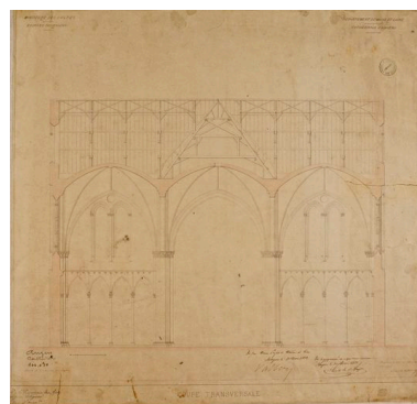
Coupe transversale à la croisée du transept, vers l'est, par Ch. Joly-Leterme, 1852. Repro. François Lasa, Autr. Charles Joly-Leterme IVR52_19934903004XA
