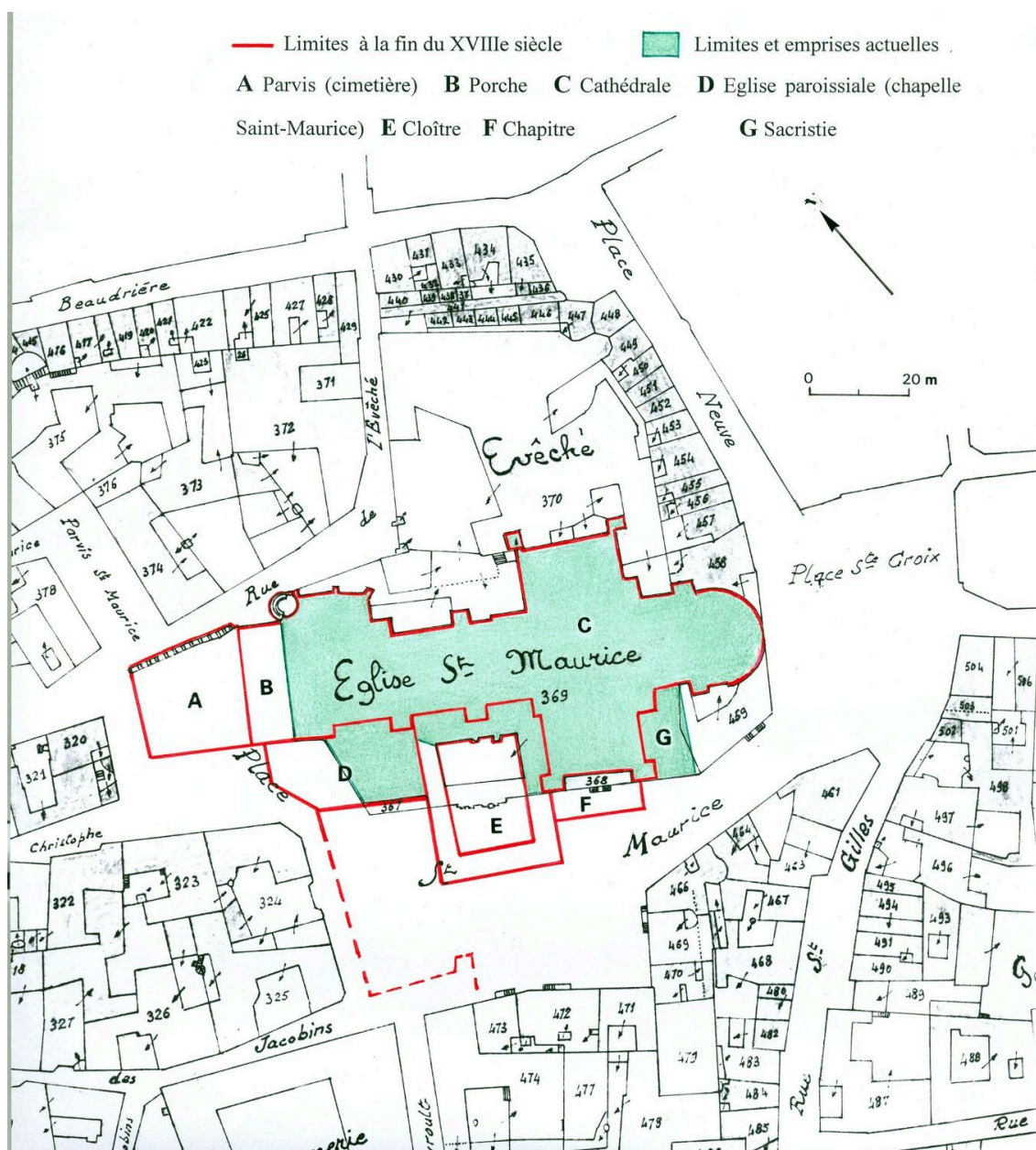
Plan-masse et de situation. D'après le plan cadastral, 1840, section J, parcelle 369, éch. 1 : 1 000.
