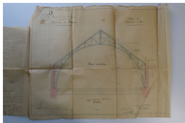
Premier projet, non réalisé, par Abel Filuzeau, 1er juin 1890 : charpente métallique. Repro. Yannis Suire IVR52_20238500325NUCA
