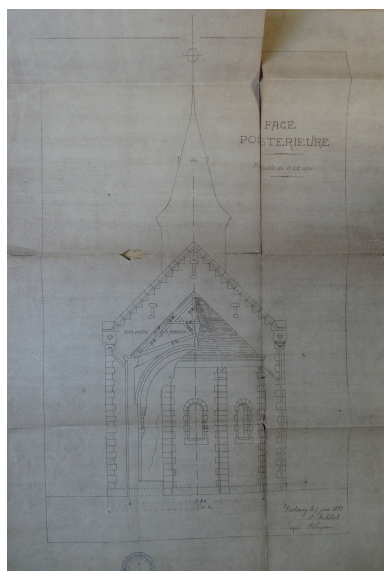
Projet par Abel Filuzeau, 5 janvier 1897 : élévation sud. Repro. Yannis Suire IVR52_20238500321NUCA
