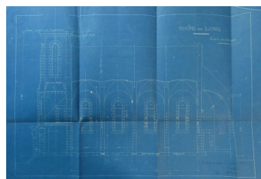
Projet par Abel Filuzeau, 5 janvier 1897 : coupe en long. Repro. Yannis Suire IVR52_20238500327NUCA
