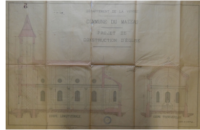
Premier projet, non réalisé, par Abel Filuzeau, 1er juin 1890 : coupes. Repro. Yannis Suire IVR52_20238500323NUCA
