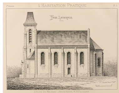
Plans de l'église du Mazeau par Abel Filuzeau, publiés dans L'Habitation pratique en avril 1899 : élévation ouest. Repro. Yannis Suire IVR52_20238500472NUCA
