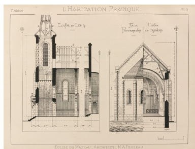
Plans de l'église du Mazeau par Abel Filuzeau, publiés dans L'Habitation pratique en avril 1899 : coupes. Repro. Yannis Suire IVR52_20238500473NUCA
