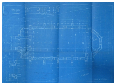
Projet par Abel Filuzeau, 5 janvier 1897 : plan. Repro. Yannis Suire IVR52_20238500319NUCA
