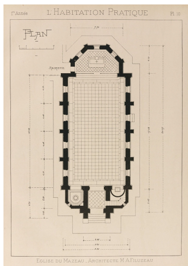
Plans de l'église du Mazeau par Abel Filuzeau, publiés dans L'Habitation pratique en avril 1899 : plan. Repro. Yannis Suire IVR52_20238500474NUCA
