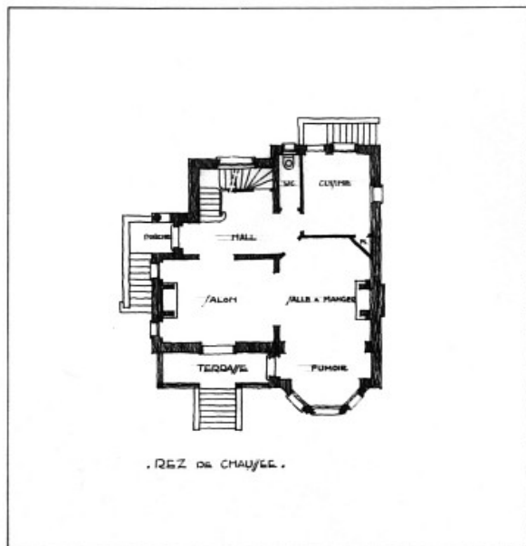
Plans d'étage et de rez-de-chaussée de la villa anglo-normande La Glorita de M. Gauthier.
