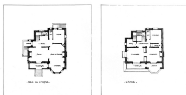
Plans d'étage et de rez-de-chaussée de la villa anglo-normande La Glorita de M. Gauthier. Autr. Adrien Grave, Phot. Denis Pillet IVR52_19984400610X
