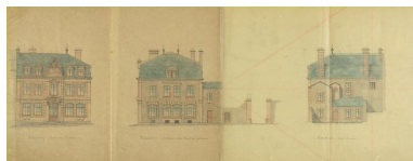
Elévations par Bordelais, en 1898. Autr. Emile II Bordelais, Phot. Patrice (reproduction) Giraud IVR52_20068500142NUCA
