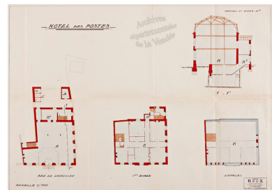
Plans et coupe de la poste au 1/100e par le cabinet Roux, vers 1930. Autr. Roux, Phot. Patrice (reproduction) Giraud IVR52_20118500393NUCA
