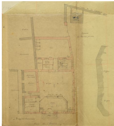
Plan du rez-de-chaussée par Bordelais, en 1898. Autr. Emile II Bordelais, Phot. Patrice (reproduction) Giraud IVR52_20068500145NUCA
