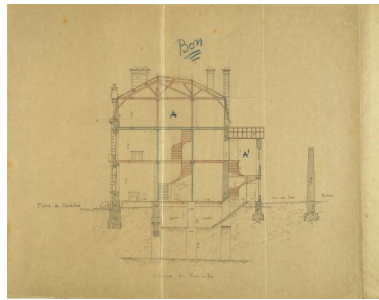
Coupe nord-sud par Bordelais, en 1898. Autr. Emile II Bordelais, Phot. Patrice (reproduction) Giraud IVR52_20068500146NUCA
