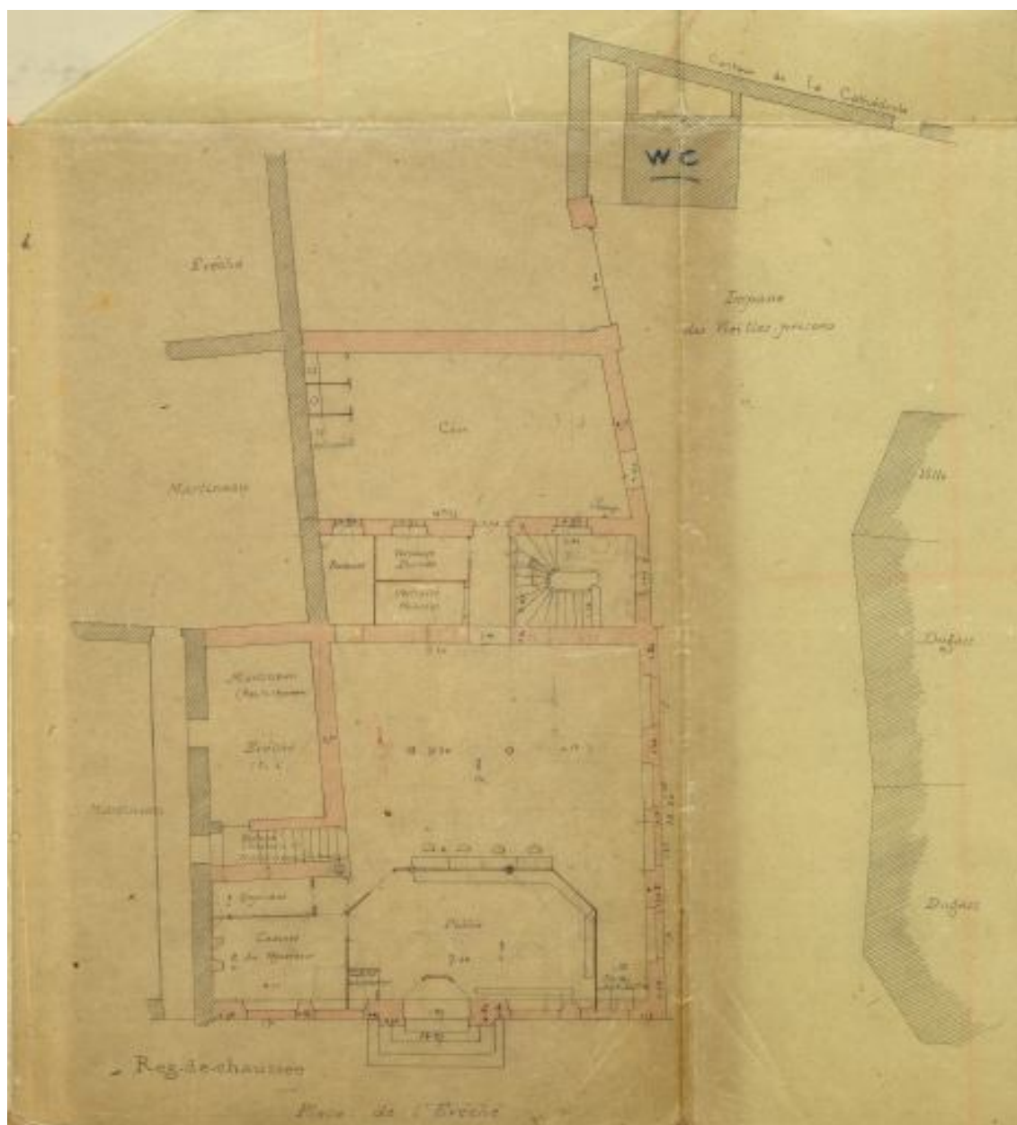
Plan du rez-de-chaussée par Bordelais, en 1898.
