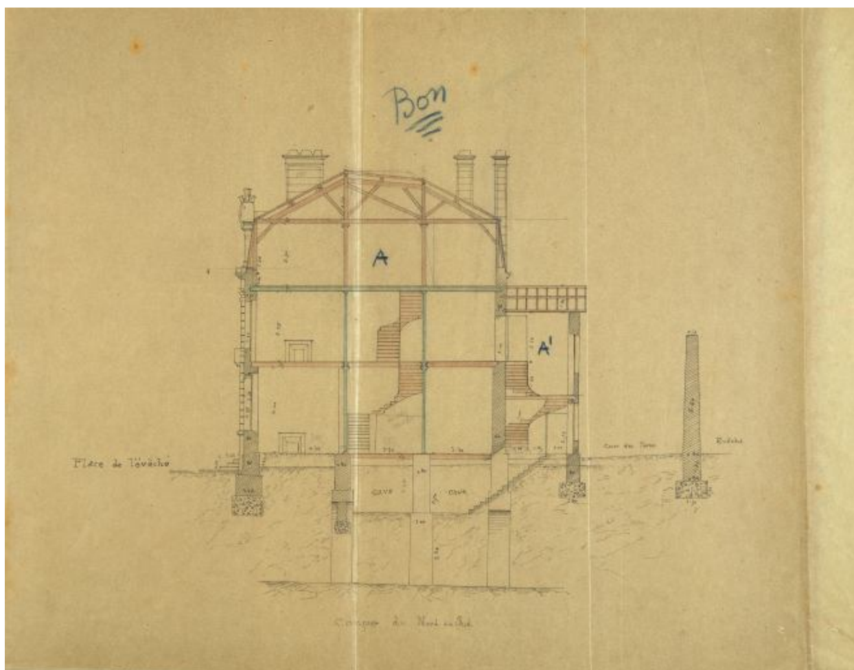
Coupe nord-sud par Bordelais, en 1898.
