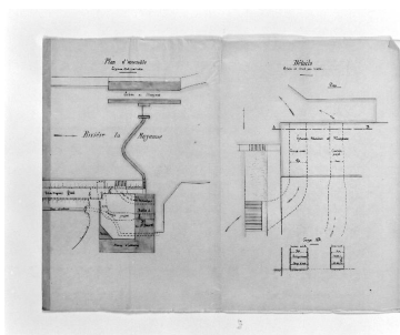
Plan d'ensemble du site d'écluse et du moulin ; plan de détail et coupe des coursiers . Autr. A. Simonet, Repro. François Lasa IVR52_20015300404X
