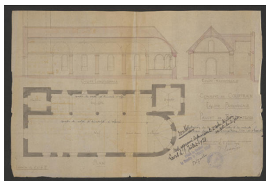
Les plans de l'église dressés par l'architecte Jules Tessier à l'occasion de la reconstruction des voûtes en 1921. Repro. Morgane Acou-Le Noan IVR52_20215300518NUCA
