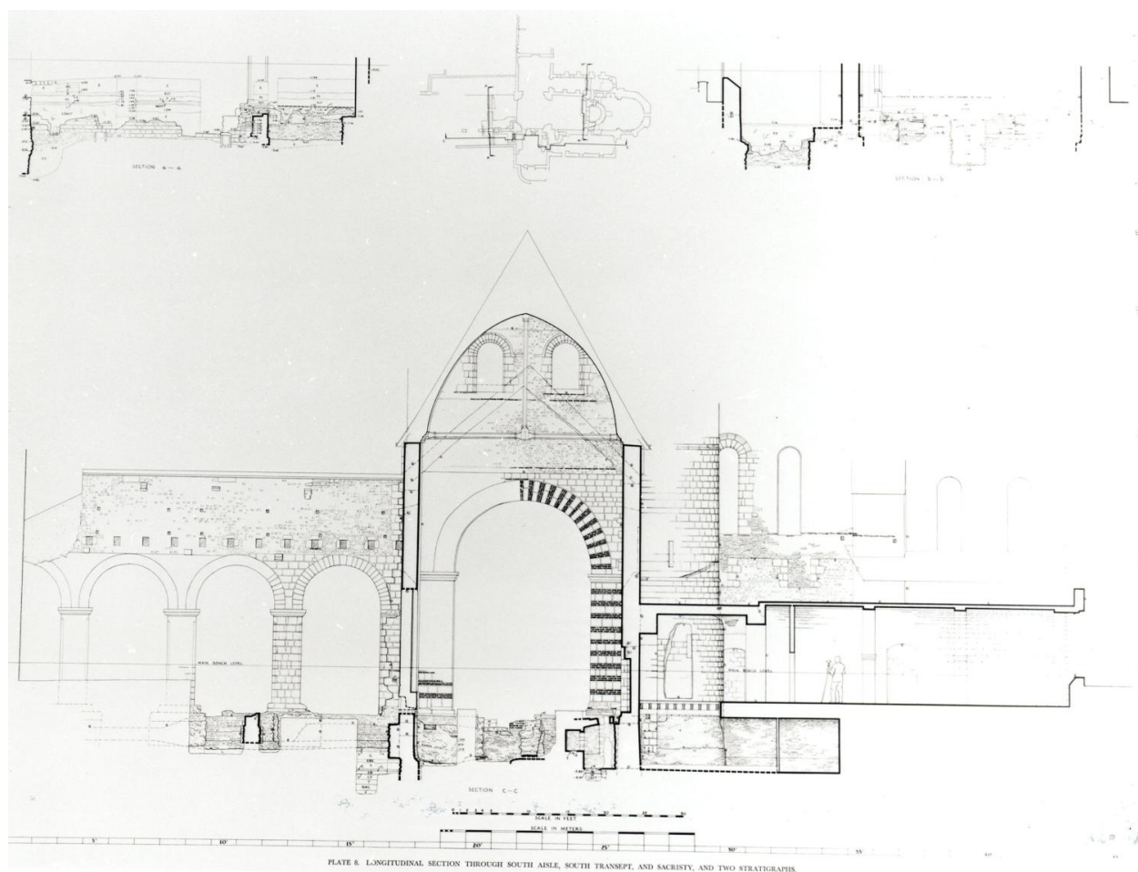
Abbatiale, coupe longitudinale, sur bas-côté sud, bras sud, 1953. Dessin, in : FORSYTH, George H, The church of St. Martin at Angers, Princeton, University Press, 1953, planche VIII.
