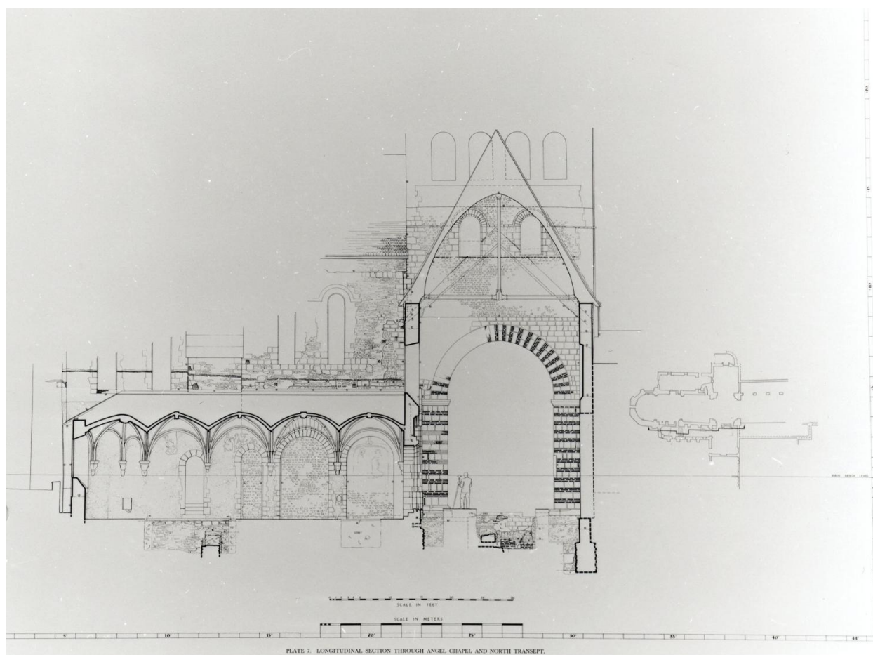
Abbatiale, coupe longitudinale, chapelle des anges et bras nord du transept, 1953. Dessin, in : FORSYTH, George H, The church of St. Martin at Angers, Princeton, University Press, 1953, planche VII.
