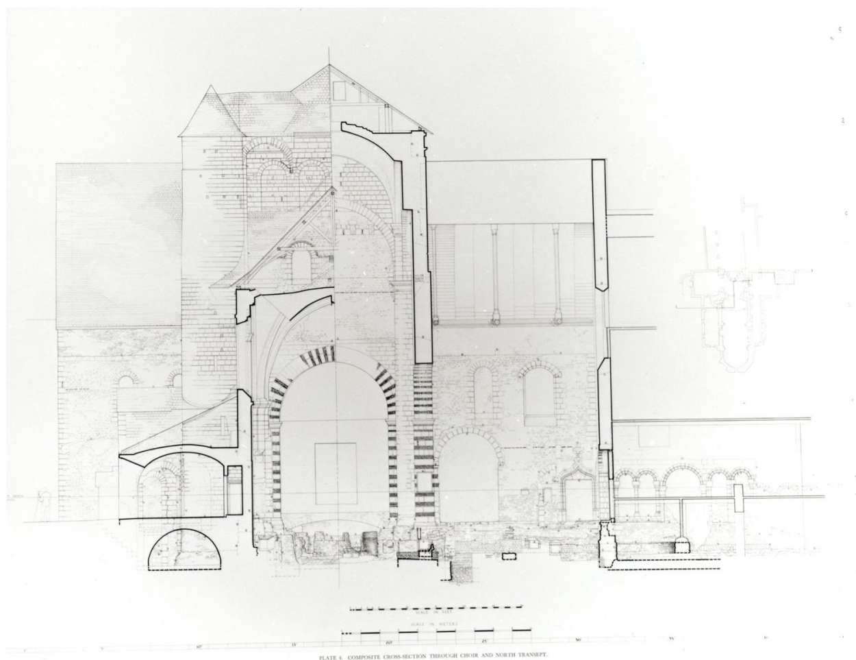
Abbatiale, coupe transversale chœur et transept, 1953. Dessin, in : FORSYTH, George H, The church of St. Martin at Angers, Princeton, University Press, 1953, planche IV.
