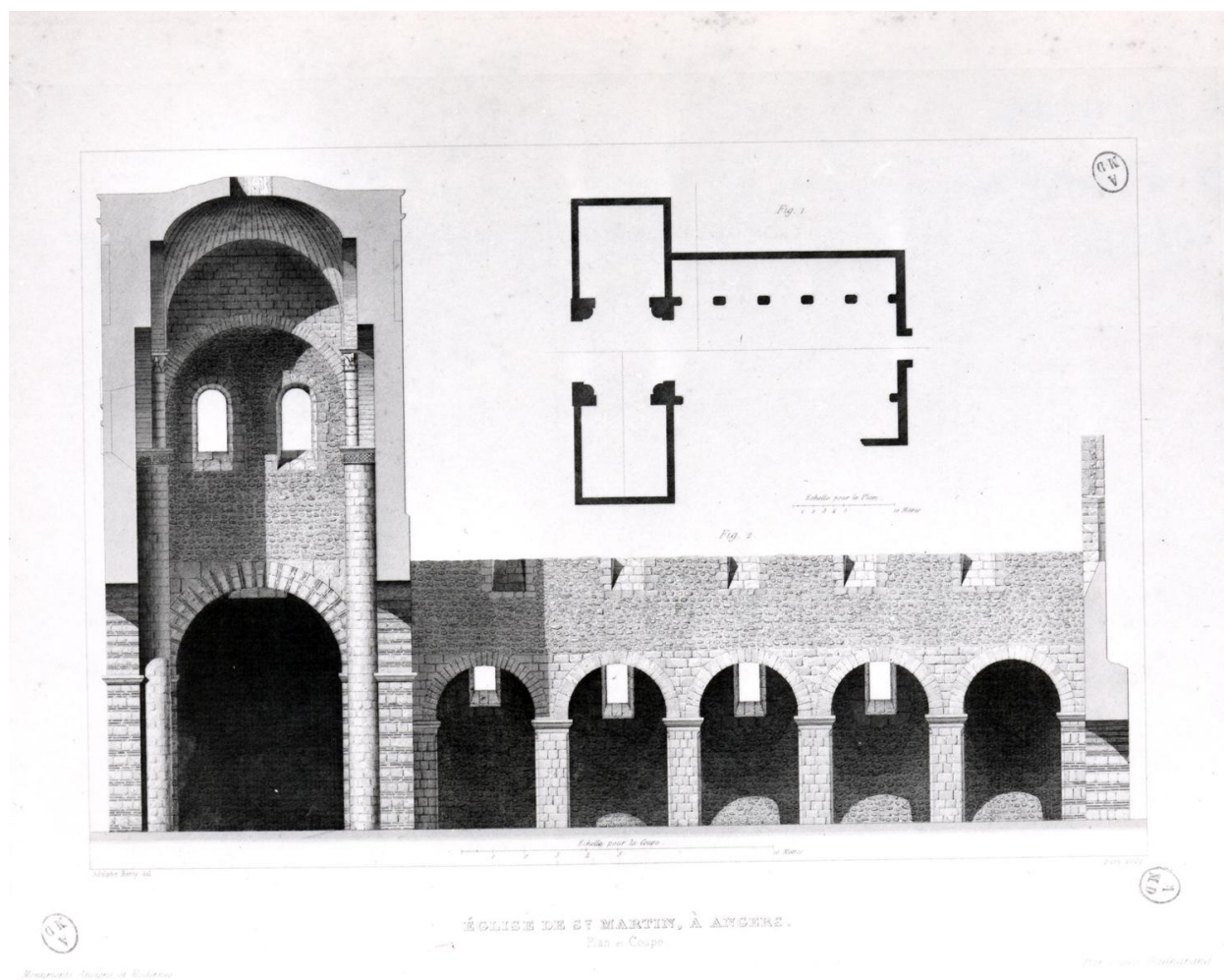
Eglise de Saint-Martin à Angers : plan et coupe, lithogr., par A. Berthy, 1847.
