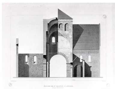
Coupe transversale de l'église, lithogr., par A. Berthy, 1847. Repro. Patrice Giraud, Repro. François Lasa IVR52_19794900583X
