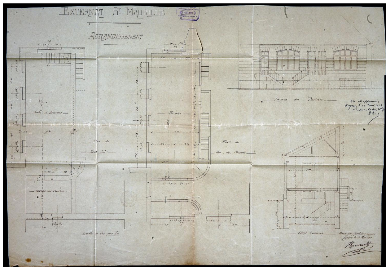
Conciergerie, plan des deux niveaux, élévation sud et coupe transversale du corps principal, projet d'agrandissement, par Félix-Joseph Ruault, 1913.
