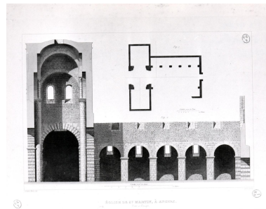
Eglise de Saint-Martin à Angers : plan et coupe, lithogr., par A. Berthy, 1847. Repro. Patrice Giraud, Repro. François Lasa IVR52_19794900585X
