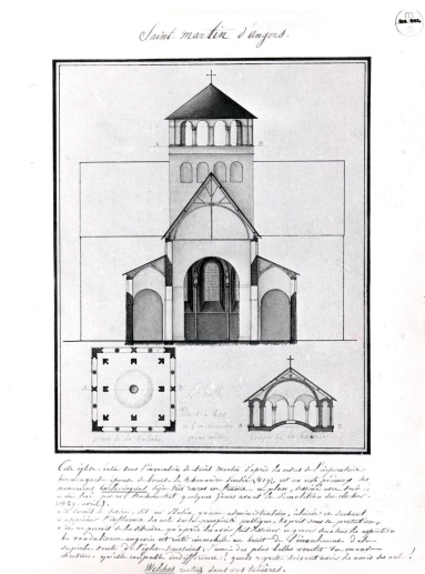
Saint-Martin d'Angers, coupe de l'église devant la tour bâtie sur la croisée du transept, par Duchouchet, 1829. Repro. Patrice Giraud, Repro. François Lasa IVR52_19794900587X
