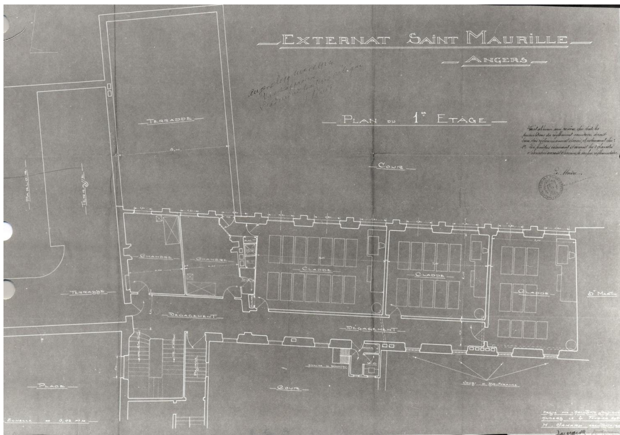
Bâtiment de classes des "moyens" et préau attenant : plan du 1er étage, par Henri Jamard, 1924.
