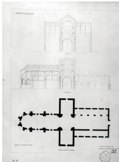
Collégiale : plan, coupes longitudinale et transversale, par Ch. Joly-Leterme, 1845. Repro. François Lasa IVR52_19934903001X
