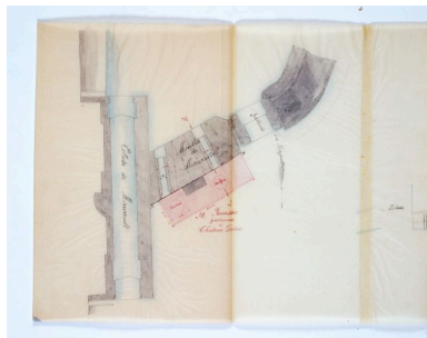
Projet d'installation de deux turbines. Plan au sol du moulin et de son extension.
