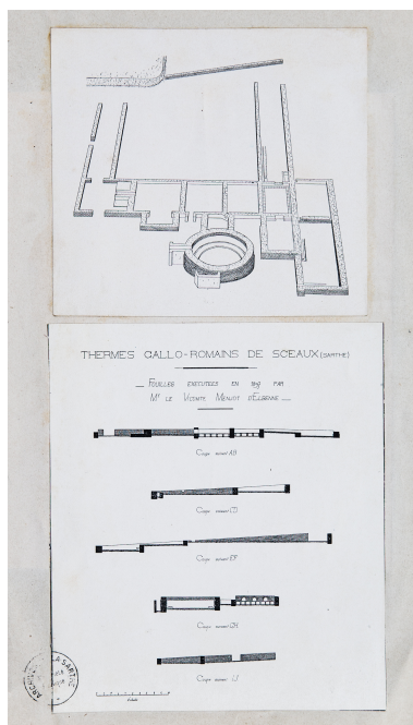
Le plan des thermes et coupes, fin du XIXe siècle. Phot. Pierre-Bernard Fourny, Autr. Samuel Menjot d'Elbenne IVR52_20187202594NUCA
