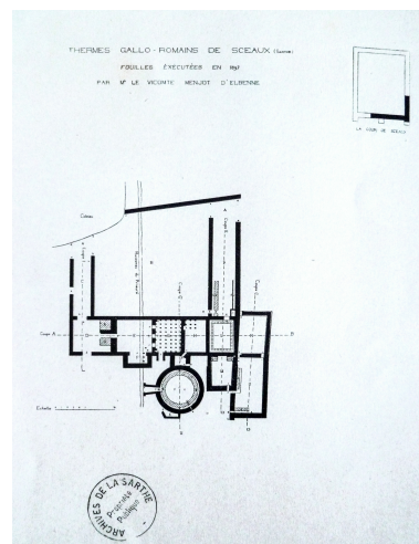
Le plan des thermes, fin du XIXe siècle. Phot. Pierre-Bernard Fourny, Autr. Samuel Menjot d'Elbenne IVR52_20187202634NUCA
