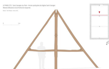
Le Mans (72) - Saint-Georges-du-Plain - Relevé d'une ferme de charpente de l'ancien presbytère de l'église Saint-Georges. Dess. Théo Ben Makhad IVR52_20217200002NUDA
