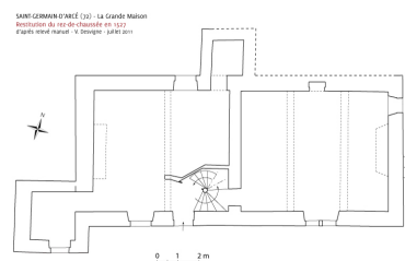
Plan du rez-de-chaussée, restitution par Christine Toulhier. Dess. Virginie Desvigne IVR52_20147202101NUDA
