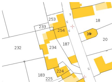
Plan en 2008. IVR52_20087210363NUCA
