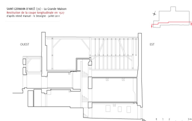
Coupe longitudinale, restitution par Christine Toulhier. Dess. Virginie Desvigne IVR52_20147202102NUDA
