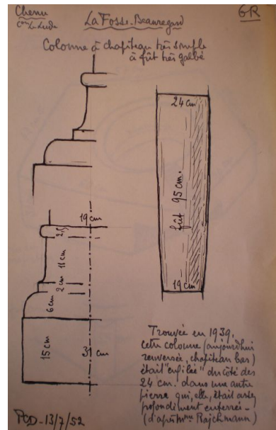
Relevé de quelques éléments d'architecture gallo-romaine. Autr. Paul Cordonnier-Détric IVR52_20087210313NUCA
