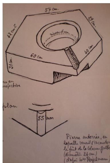
Relevés de quelques éléments d'architecture gallo-romaine. Autr. Paul Cordonnier-Détré IVR52_20087210314NUCA
