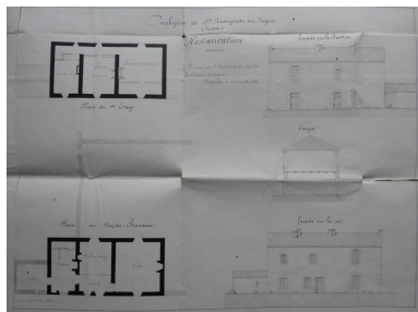
Plans et élévations de l'ancien presbytère, 15 novembre 1860. Phot. Yannis (reproduction) Suire IVR52_20188501119NUCA
