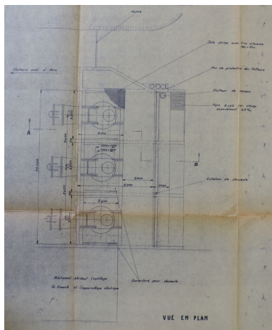
Projet de station de pompage par le Génie rural, 5 novembre 1964 : plan. Phot. Yannis Suire IVR52_20228501228NUCA
