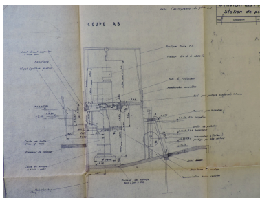
Projet de station de pompage par le Génie rural, 5 novembre 1964 : coupe. Phot. Yannis Suire IVR52_20228501207NUCA
