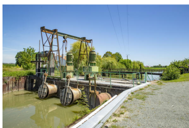
Les pompes de la Grande cabane. Phot. Pierre-Bernard Fourny IVR52_20208501280NUCA
