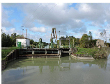
Le barrage vu depuis l'amont, à l'est.
