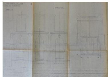
Projet de station de pompage par le Génie rural, 5 novembre 1964 : élévation amont. Phot. Yannis Suire IVR52_20228501185NUCA
