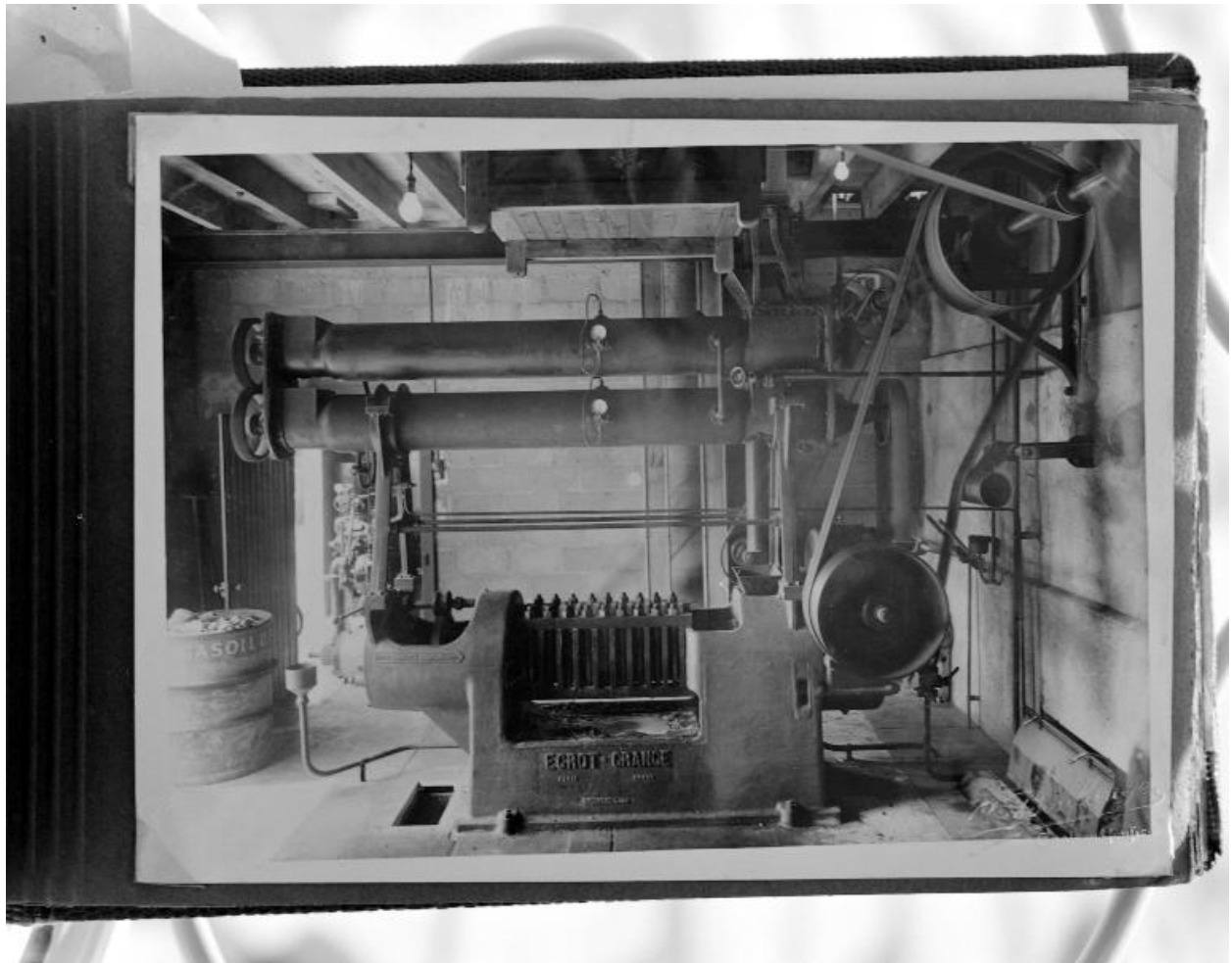
Le bâtiment de raffinage, dit "usine à arachide", en 1934 (?). Vue intérieure : la presse hydraulique à arachide.
