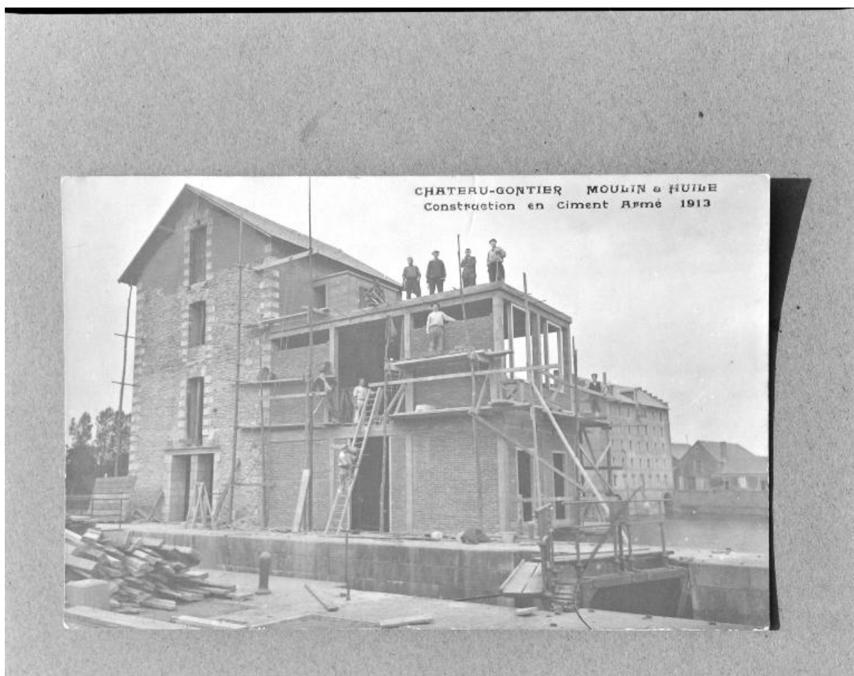
Le moulin vu du sud-ouest lors de la construction de l'extension en béton et en brique, en 1913.
