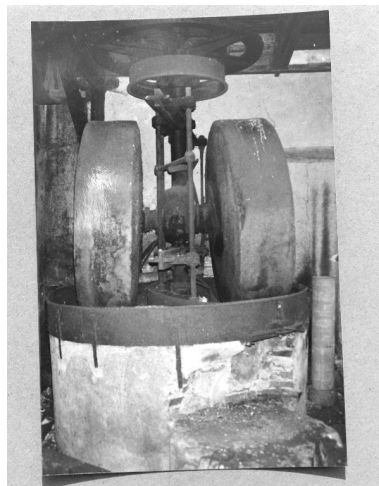
Premier étage du moulin : les meules à huiles avant la destruction du moulin, en 1991. Repro. François Lasa IVR52_20025300630X
