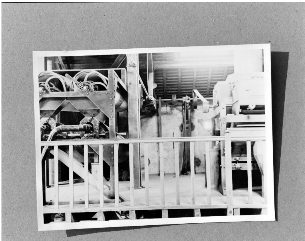
Le bâtiment de stockage, en 1931. Vue intérieure. Le système de nettoyage des grains vu de face. A gauche, la table de nettoyage.
