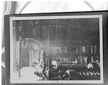
Les presses à arachide nouvellement installées, en 1938. Repro. François Lasa IVR52_20025300648X
