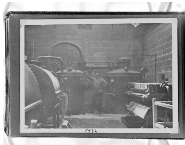
Le bâtiment de raffinage, en 1934. Vue intérieure. A gauche, le neutralisateur et le décolorateur. Au fond, le désodoriseur et le refroidisseur. A droite, le filtre-plaque.
