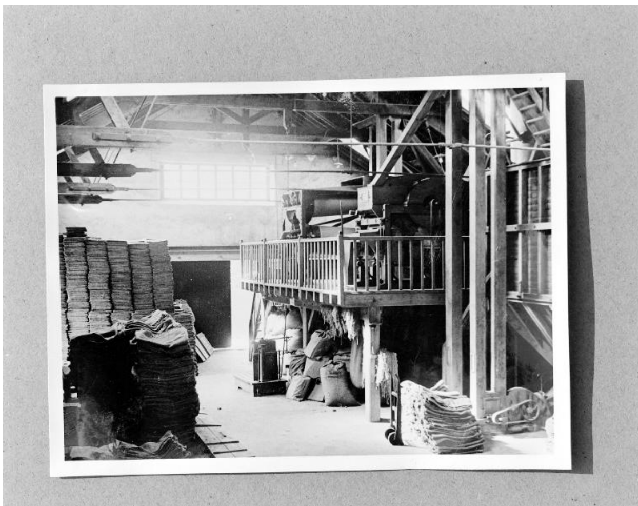
Le bâtiment de stockage, en 1931. Vue intérieure. A droite, le système de nettoyage des graines.
