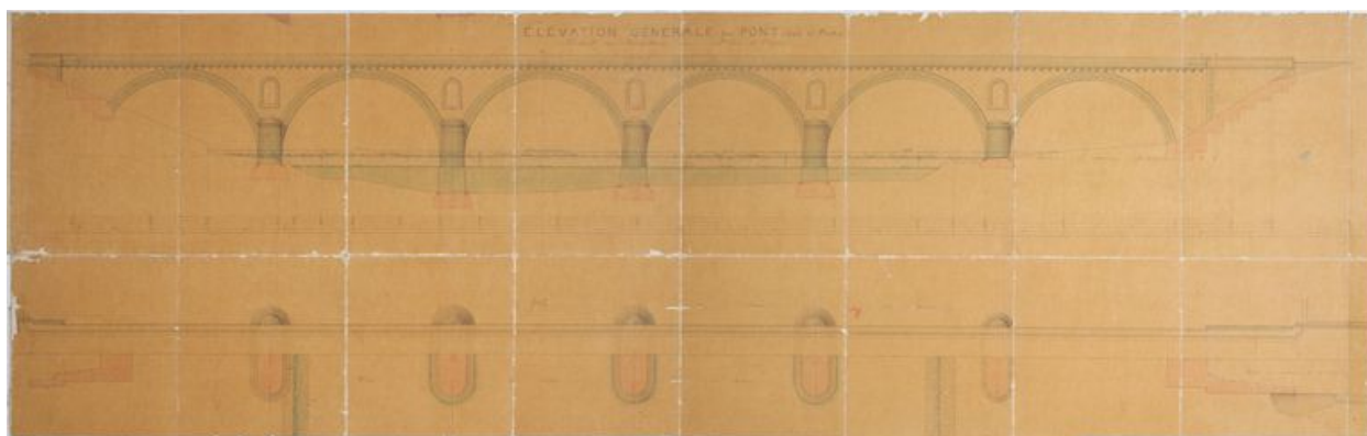
Elévation et plan du pont.
