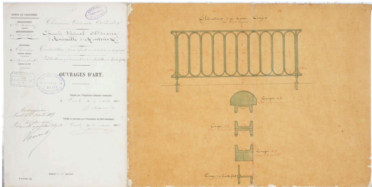
Elévation et coupes des garde-corps du pont.
