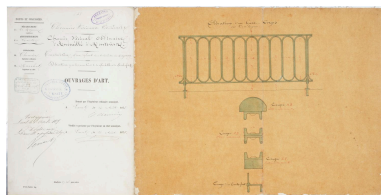
Elévation et coupes des garde-corps du pont. Repro. Yves Guillotin, Autr. Chemin IVR52_20095300155NUCA
