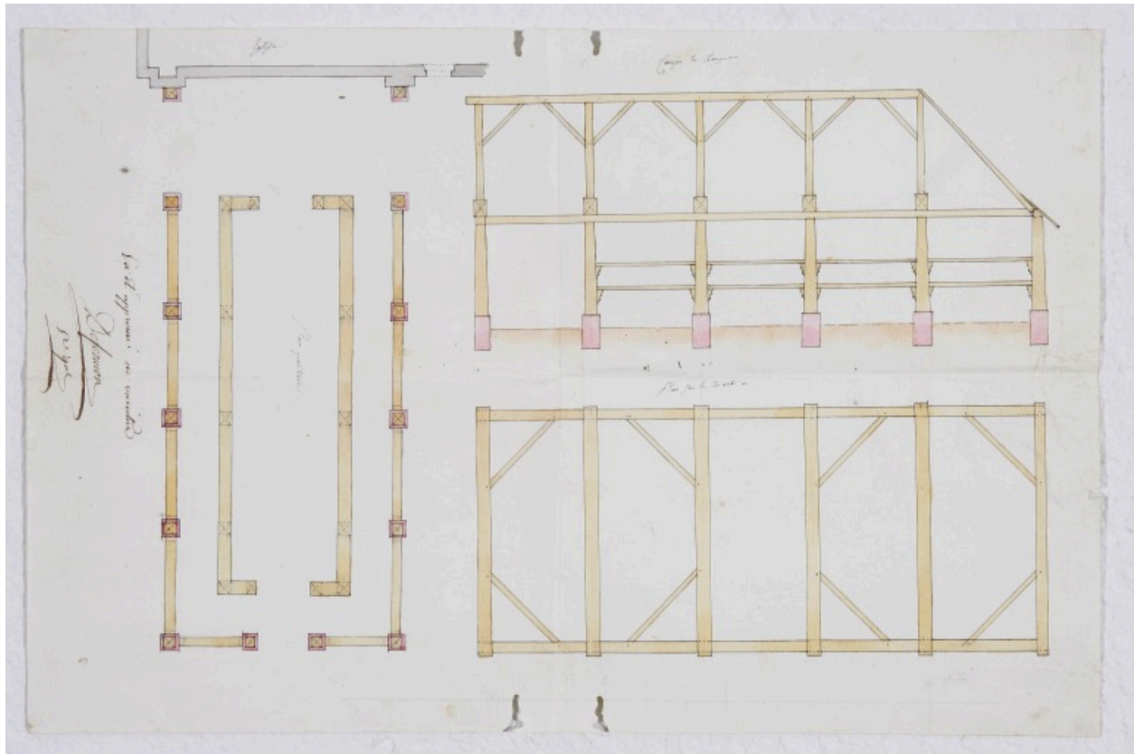
Projet de construction de la halle, vers 1803 : plan au sol, plan au niveau des tirants et coupe longitudinale.
