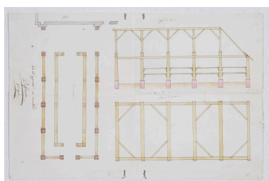
Projet de construction de la halle, vers 1803 : plan au sol, plan au niveau des tirants et coupe longitudinale. Repro. François Lasa IVR52_20045303469NUCA
