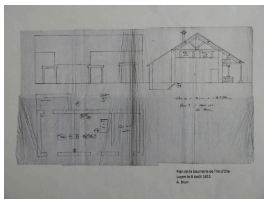
Plan de la beurrerie, par A. Brun, 9 août 1911.
