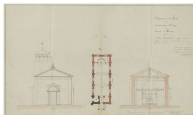
2e projet d'église pour Damvix, par Auguste Garnereau, 16 avril 1848 (projet rejeté) : élévation ouest, plan et coupe transversale. Phot. Yannis (reproduction) Suire, Autr. Auguste Garnereau IVR52_20228501050NUCA
