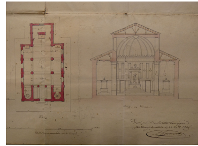
Premier projet de construction d'une nouvelle église à Damvix par Auguste Garnereau, 22 décembre 1845 : plan et coupe. Phot. Yannis (reproduction) Suire, Autr. Auguste Garnereau IVR52_20228501101NUCA
