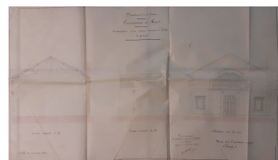
Projet de préau par Abel Filuzeau, 1886. Repro. Yannis Suire IVR52_20238502303NUCA
