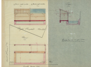
Lavoir communal de Saint-Georges-de-la-Couée : plan au sol, coupe et élévation, 1901. Repro. Pierre-Bernard Fourny IVR52_20267200030NUCA
