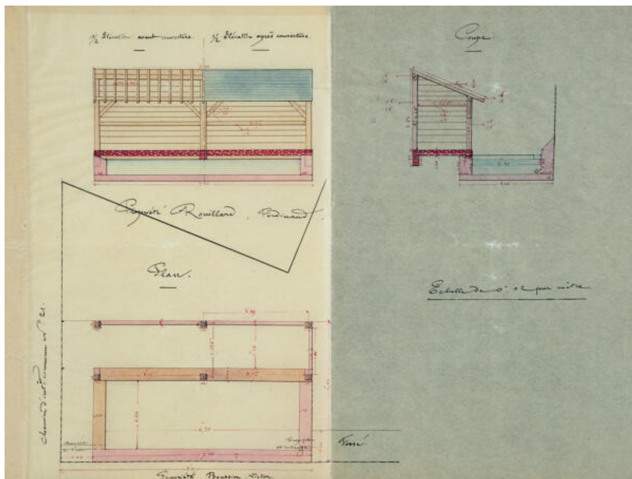
Lavoir communal de Saint-Georges-de-la-Couée : plan au sol, coupe et élévation, 1901.
