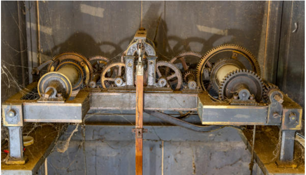
Vue du mécanisme de l'horloge de l'église Notre-Dame.
