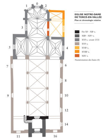
Plan de l'église Notre-Dame, 2015. Phot. Jérôme Bulard IVR52_20217201554NUCA
