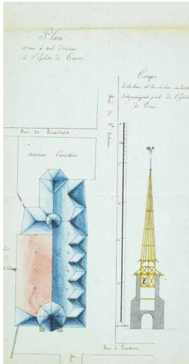
Plan et coupe de l'église et de son clocher, 1816.
