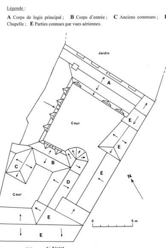
Plan schématique de couverture pour l'état avant la fin des années 1970. Dess. I. Frager IVR52_20004904533A4
