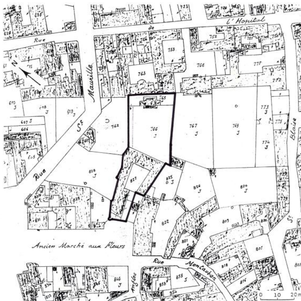
Plan-masse et de situation. D'après le plan cadastral, 1840, section H2, parcelles 765, 766, 827, éch. 1 : 1 000.
