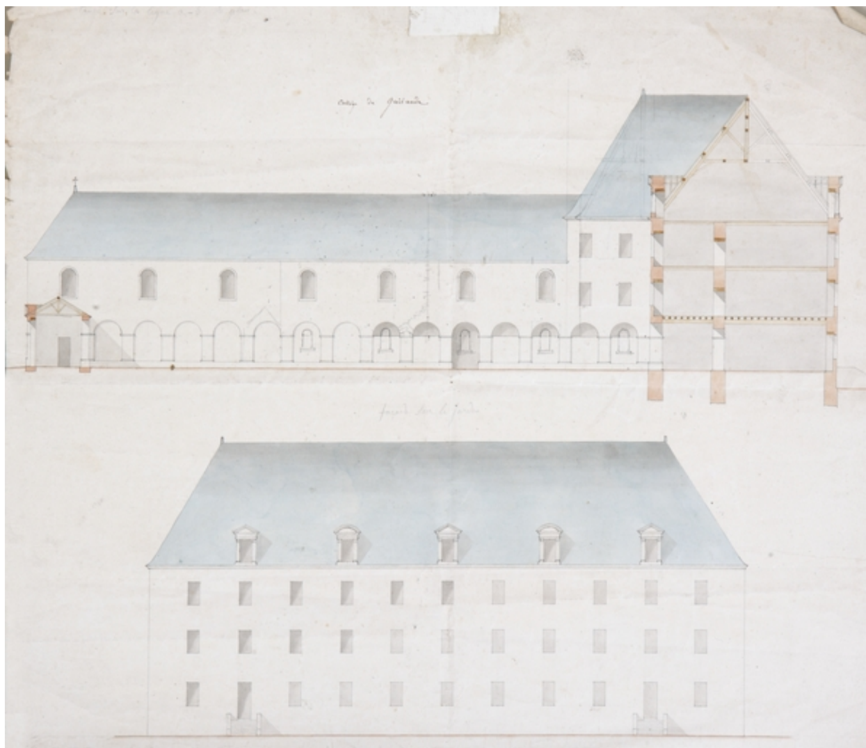
Elévation et coupe de l'aile nord par Henri Gilée, architecte, 2e moitié XIXe siècle.
