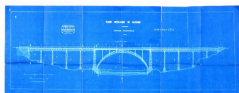
Projet, presque définitif, du 25 septembre 1900. Elévation. Autr. Moisant, Laurent, Savey et Cie, Phot. François (reproduction) Lasa IVR52_20025300478XA
