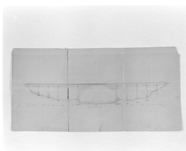
Projet du 13 juillet 1899, adoptant le système Hennebique de construction en béton de ciment armé. Elévation. Phot. François (reproduction) Lasa IVR52_20025300485X
