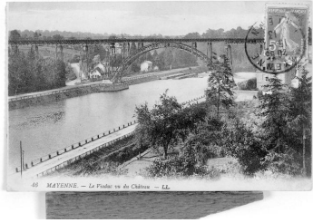
Vue d'ensemble du viaduc depuis la rive droite, en amont de la rivière. Phot. François (reproduction) Lasa IVR52_20015300368XB
