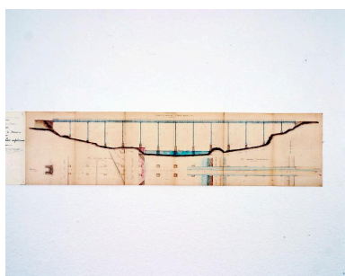
Projet du 21 octobre 1899. Elévation et plan. Autr. L. Verrier, Phot. François (reproduction) Lasa IVR52_20025300482XA
