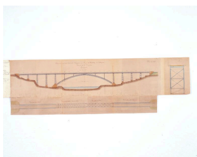
Projet du 10 août 1898. Elévation, plan, coupe transversale. Phot. François (reproduction) Lasa IVR52_20025300476XA
