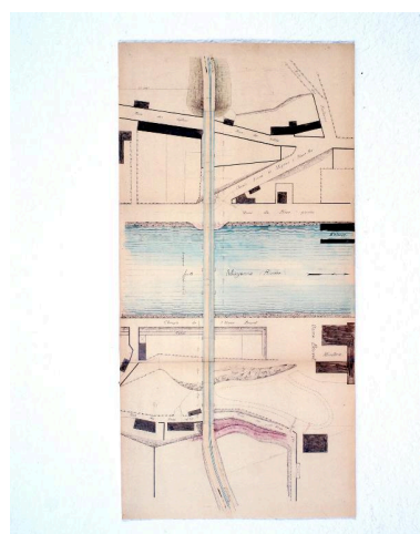
Projet du 21 octobre 1899. Plan et localisation. Autr. L. Verrier, Phot. François (reproduction) Lasa IVR52_20025300484XA
