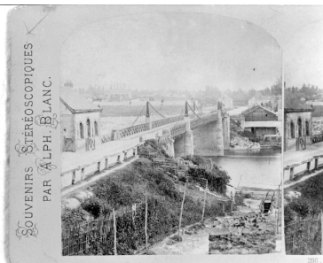
Vue d'ensemble du pont suspendu, construit en 1842, reconstruit en 1848 et abattu en 1872. Autr. Alphonse Blanc, Phot. François (reproduction) Lasa IVR52_20035300008XB
