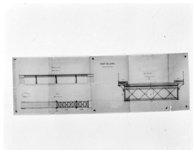
Projet non réalisé, 1870 : élévation générale, plan et coupe transversale. Autr. Gustave Eiffel, Phot. François (reproduction) Lasa IVR52_20025300329X
