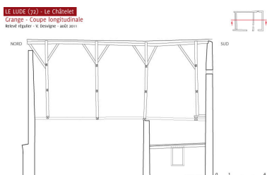
La grange, coupe longitudinale, état actuel. Dess. Virginie Desvigne IVR52_20117200112NUDA
