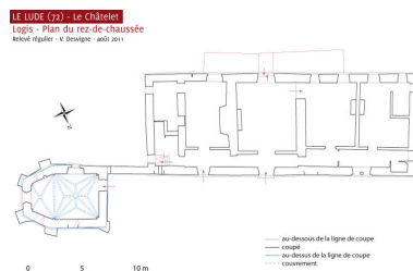
Plan du rez-de-chaussée de la maison et de la chapelle, état actuel. Dess. Virginie Desvigne IVR52_20117200107NUDA
