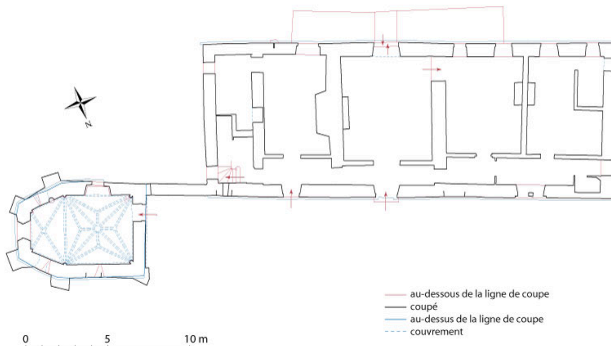
Plan du rez-de-chaussée de la maison et de la chapelle, état actuel.
