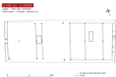
Plan du comble, état actuel. Dess. Virginie Desvigne IVR52_20117200108NUDA
