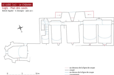
Plan du sous-sol de la maison et de la chapelle, état actuel. Dess. Virginie Desvigne IVR52_20117200106NUDA
