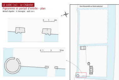
Plan de situation des différentes constructions situées sur la plateforme. Dess. Virginie Desvigne IVR52_20117200104NUDA
