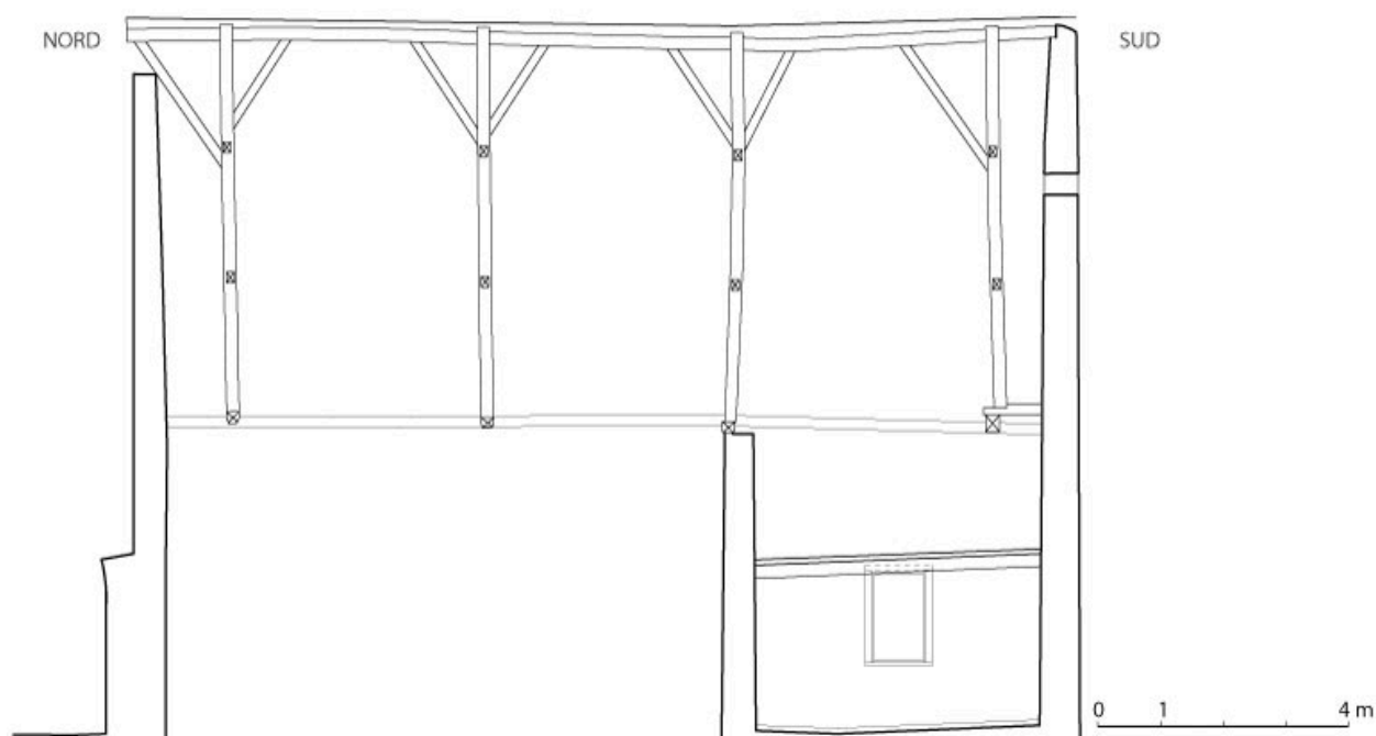
La grange, coupe longitudinale, état actuel.
