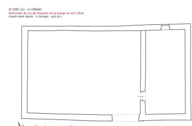
La grange, restitution du plan (1522). Dess. Virginie Desvigne, Dess. Christine Toulhier IVR52_20147202105NUDA
