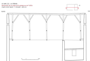
La grange, restitution de la coupe longitudinale. Dess. Virginie Desvigne IVR52_20147202106NUDA
