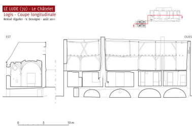
Coupe longitudinale de la maison et de la chapelle, état actuel. Dess. Virginie Desvigne IVR52_20117200109NUDA
