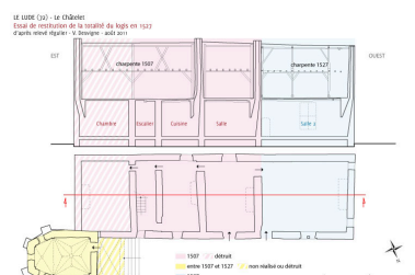
Essai de restitution des phases de construction du logis et de la chapelle entre 1507 et 1527, par Christine Toulhier. Dess. Virginie Desvigne, Dess. Christine Toulhier IVR52_20147202097NUDA
