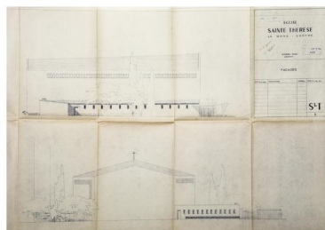
Elévation des façades est et postérieure. Repro. Bruno Rousseau, Autr. Pierre Vago IVR52_20217200271NUCA
