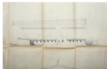
Elévation de la façade latérale est (détail). Repro. Bruno Rousseau IVR52_20217200272NUCA
