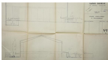
Coupe transversale (détail). Repro. Bruno Rousseau, Autr. Pierre Vago IVR52_20217200268NUCA
