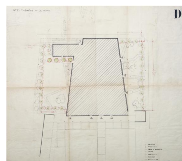
Plan masse de l'église. Repro. Bruno Rousseau, Autr. Pierre Vago IVR52_20217200264NUCA
