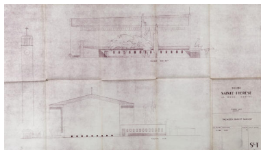
Elévations des façades sud et sud-est de l'église Sainte-Thérèse par Pierre Vago. Repro. Pierre-Bernard Fourny, Autr. Pierre Vago IVR52_20217200143NUCA
