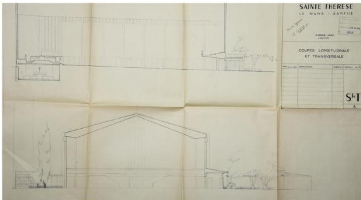
Coupe transversale (détail).
