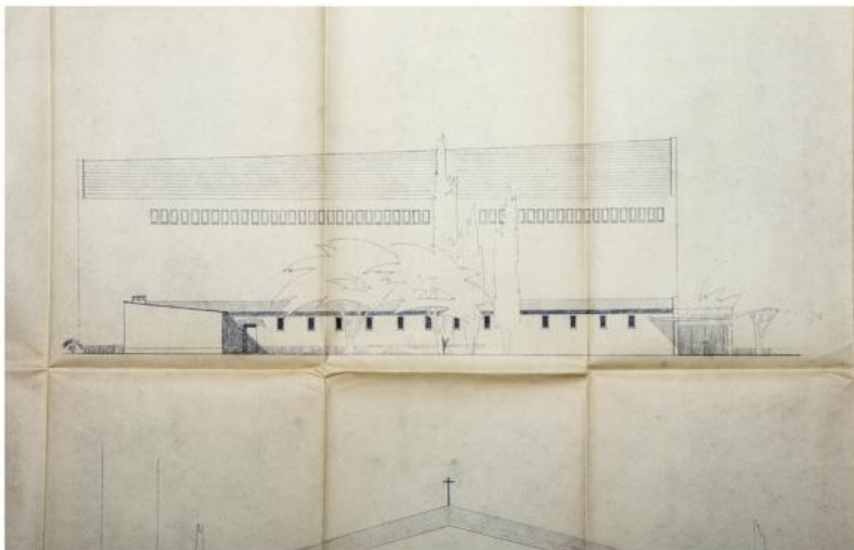
Elévation de la façade latérale est (détail).
