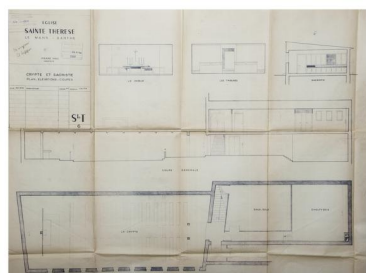
Plan, coupe et élévation de la crypte et de la sacristie. Repro. Bruno Rousseau, Autr. Pierre Vago IVR52_20217200269NUCA
