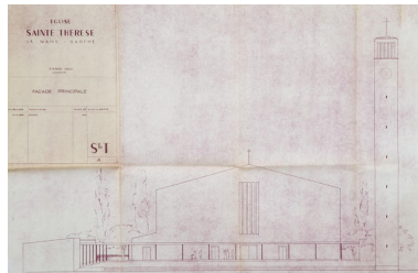
Elévation de la façade principale de l'église Sainte-Thérèse par Pierre Vago. Repro. Pierre-Bernard Fourny, Autr. Pierre Vago IVR52_20217200144NUCA
