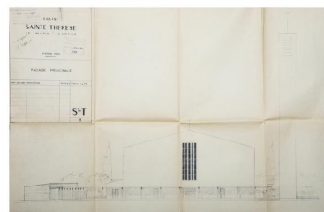
Elévation de la façade principale de l'église. Repro. Bruno Rousseau, Autr. Pierre Vago IVR52_20217200274NUCA
