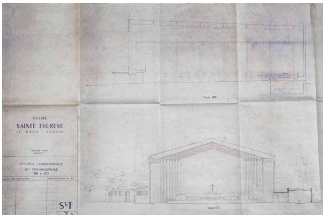
Coupes longitudinales et transversales de l'église Sainte-Thérèse par Pierre Vago.
