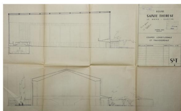
Coupes transversale et longitudinale de l'église. Repro. Bruno Rousseau, Phot. Pierre Vago IVR52_20217200266NUCA
