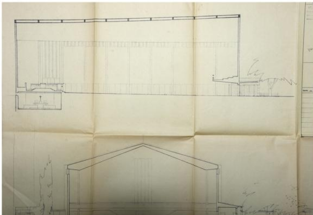
Coupe longitudinale (détail).
