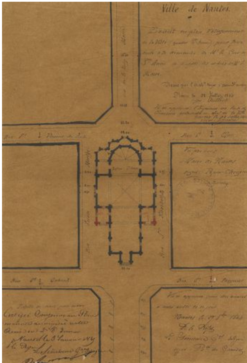
Plan de l'église Sainte-Anne, après 1872.
