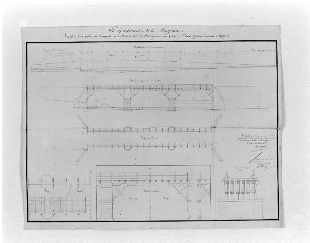
Projet de pont en bois (non réalisé), 1830. Elévations, plan, coupe transversale.
