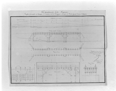
Projet de pont en bois (non réalisé), 1830. Elévations, plan, coupe transversale. Autr. Charles Collignon, Repro. François Lasa IVR52_20025300453X
