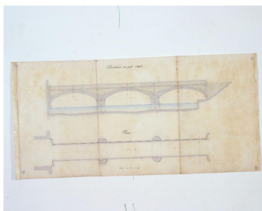
Plan et élévation sud du pont avant son exhaussement et son élargissement, 1882. Autr. A. Simonet, Repro. François Lasa IVR52_20025300148XA
