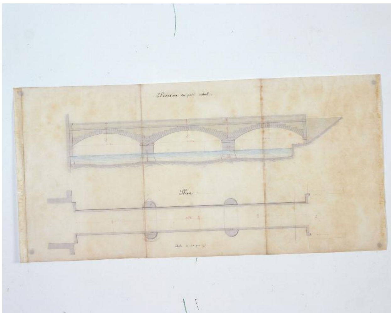
Plan et élévation sud du pont avant son exhaussement et son élargissement, 1882.
