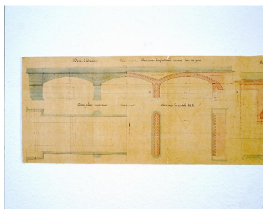
Projet de pont en pierre (non réalisé), 1830. Détail : demi- élévation, demi-plan, demi-coupes longitudinale et transversale. Autr. Charles Collignon, Repro. François Lasa IVR52_20025300452XA
