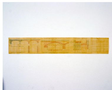
Projet de pont en pierre (non réalisé), 1830. Demi-élévation, demi- plan, demi-coupes longitudinale et transversale ; coupes du cintre nécessaire à la construction. Autr. Charles Collignon, Repro. François Lasa IVR52_20025300450XA
