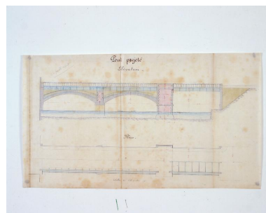
Projet (non réalisé) du 16 juin 1882 d'exhaussement et d'élargissement. Plan et élévation sud. Autr. A. Simonet, Repro. François Lasa IVR52_20025300150XA
