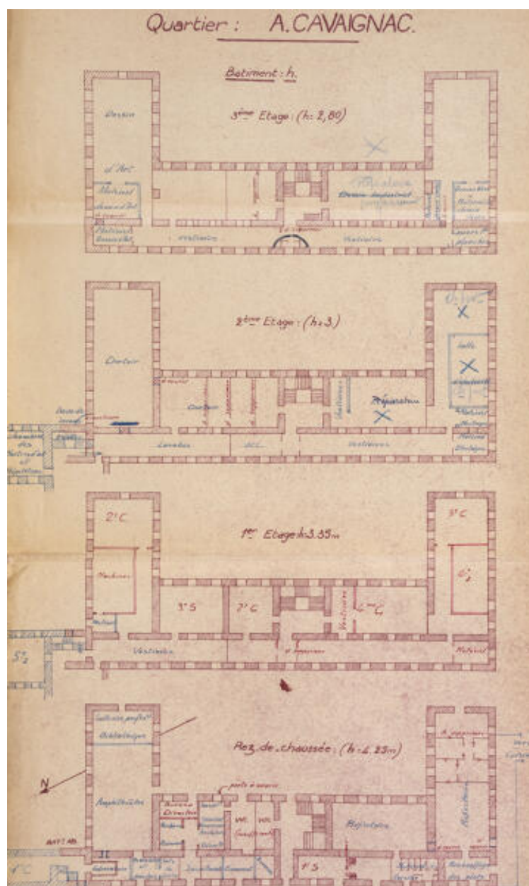
Plan du rez-de-chaussée, 1er, 2e et 3e étages du bâtiment H de la caserne Cavaignac, s.d.
