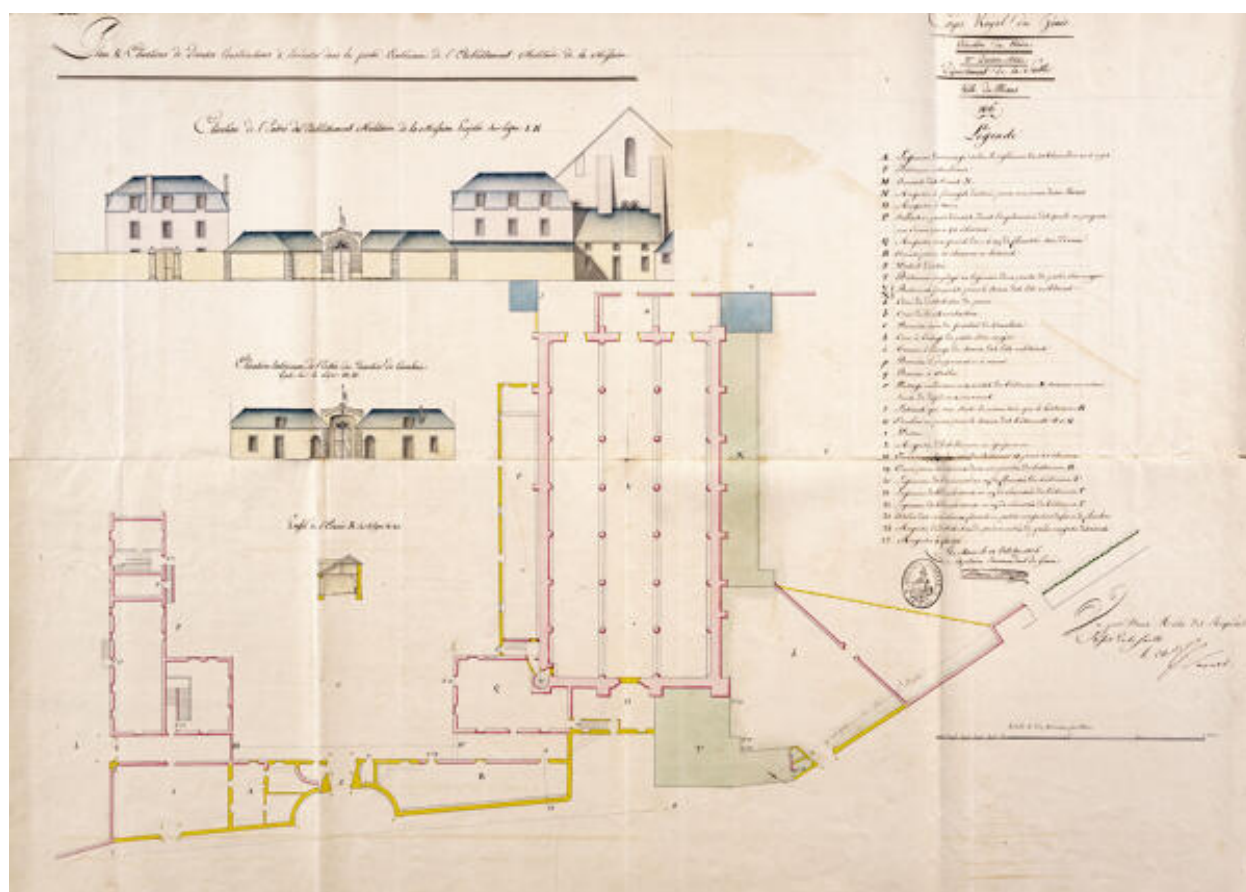
Plan et élévation des bâtiments des écuries pour l'agrandissement de la caserne Cavaignac.
