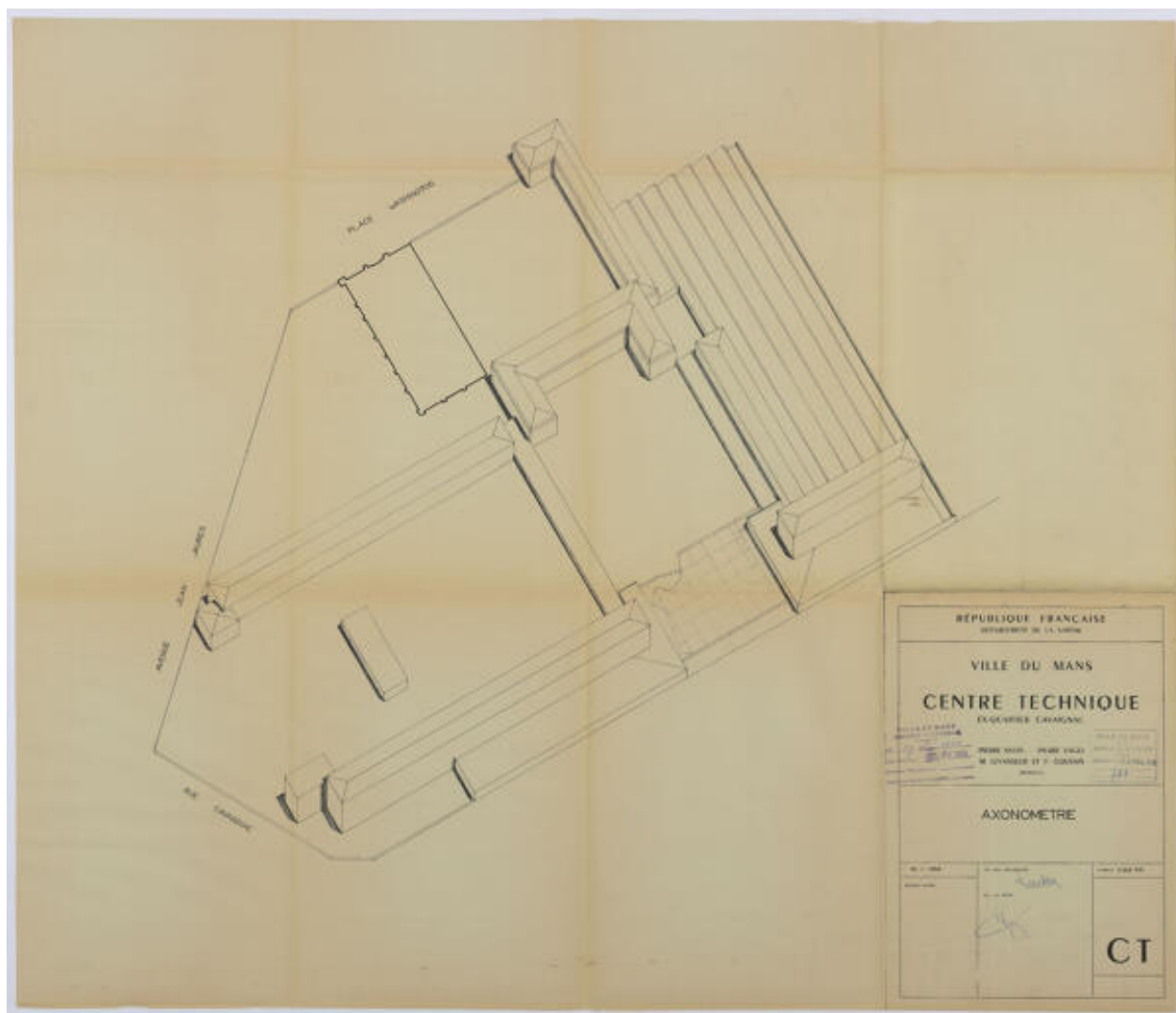
Plan axonométrique des bâtiments du centre technique.
