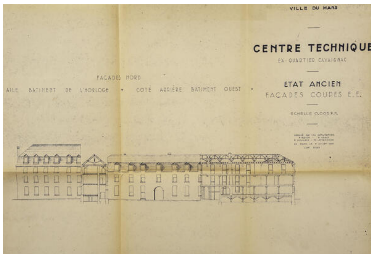
Elévation de la façade état ancien du centre technique anciennement caserne Cavaignac, 6 juillet 1948.
