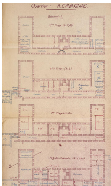
Plan et élévation des bâtiments des écuries pour l'agrandissement de la caserne Cavaignac. Repro. Pierre-Bernard Fourny IVR52_20227200449NUCA
