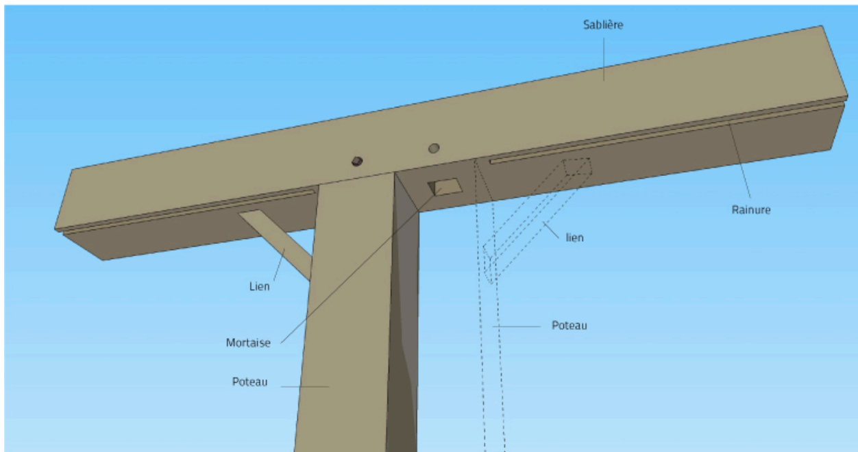
SAINT-LÉGER - L'Étarderie Ancien logis transformé en écurie DÉTAIL DE L'ASSEMBLAGE DE POTEAUX JUMELÉS AVEC LA SABLÈRE
