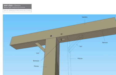
Dessin de détail du pan de bois du mur nord de l'ancien logis : assemblage de poteaux jumelés avec la sablière. Dess. Virginie Desvigne, Dess. Élodie Rama IVR52_20105300348NUDA
