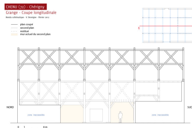
La grange : coupe longitudinale. Dess. Virginie Desvigne IVR52_20127200515NUCA
