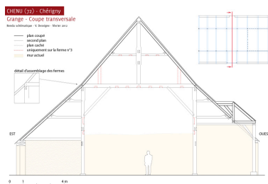
La grange : coupe transversale. Dess. Virginie Desvigne IVR52_20127200513NUDA
