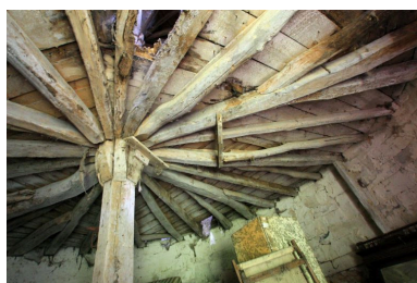
La basse-cour du château, pigeonnier : rez-de-chaussée. Phot. Jean-Baptiste Darrasse IVR52_20087201700NUCA
