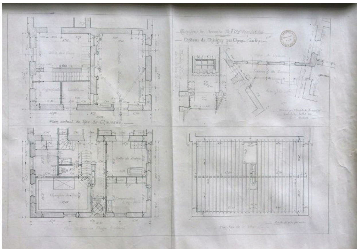
Plans de la surélévation de l'extrémité du logis côté basse-cour et construction d'une galerie de service. (Plan, 1916 ; non coté. Collection particulière).
