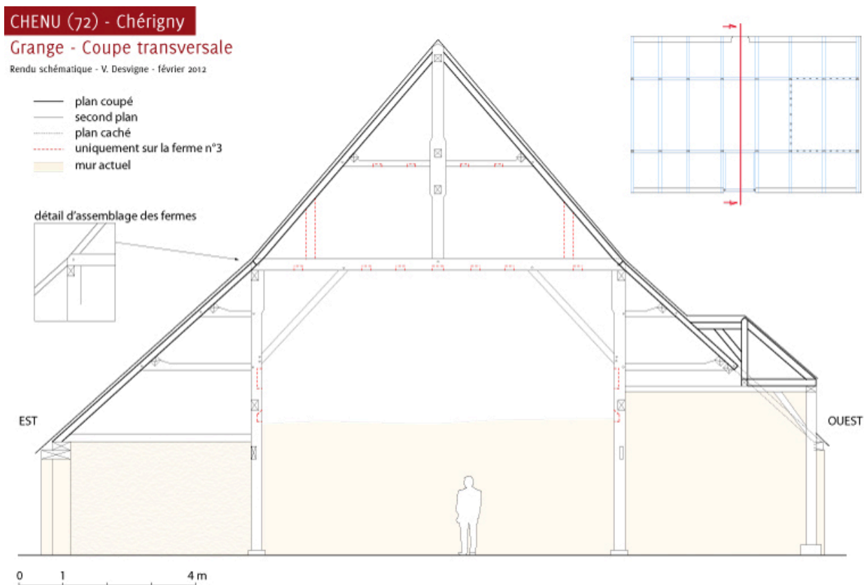
La grange : coupe transversale.
