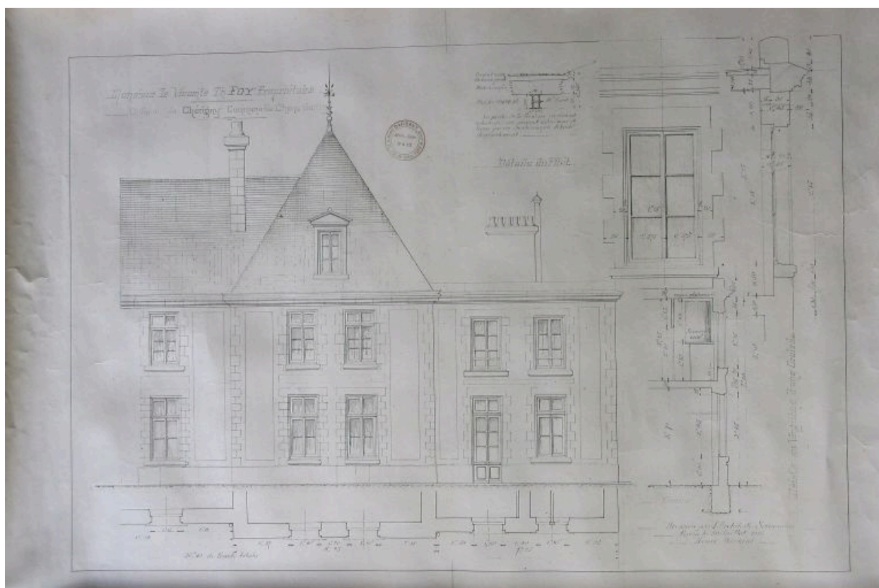
Élévation de la surélévation, 1916. (Collection particulière).
