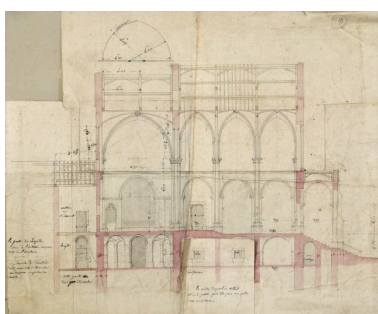
Projet Tournesac et Tessier modifié : coupe longitudinale sud-nord de l'église.
