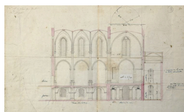
Projet Tournesac et Tessier modifié : coupe longitudinale nord-sud de l'église.
