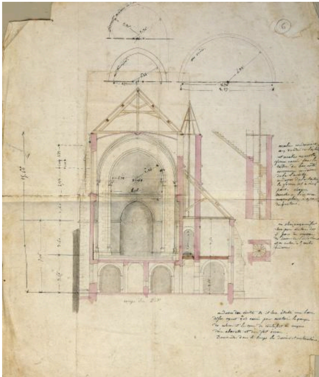
Projet Tournesac et Tessier modifié : coupe transversale de l'église.
