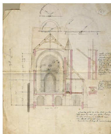
Projet Tournesac et Tessier modifié : coupe transversale de l'église. Autr. Magloire Tournesac, Autr. Alfred Tessier, Phot. Patrice (reproduction) Giraud IVR52_20068500222NUCA
