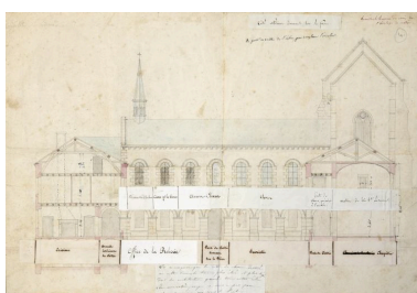
Projet Tournesac et Tessier modifié : coupe ouest-est, vers le nord. Autr. Magloire Tournesac, Autr. Alfred Tessier, Phot. Patrice (reproduction) Giraud IVR52_20068500220NUCA
