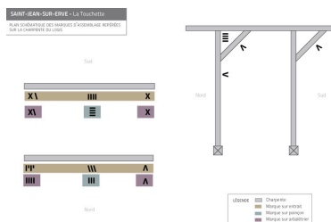
Charpente. Répartition des marques d'assemblage repérées. Dess. Élodie Rama IVR52_20105300449NUDA
