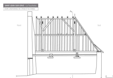
Coupe longitudinale de l'étage et du comble. Dess. Laurent Cohin IVR52_20105300421NUDA
