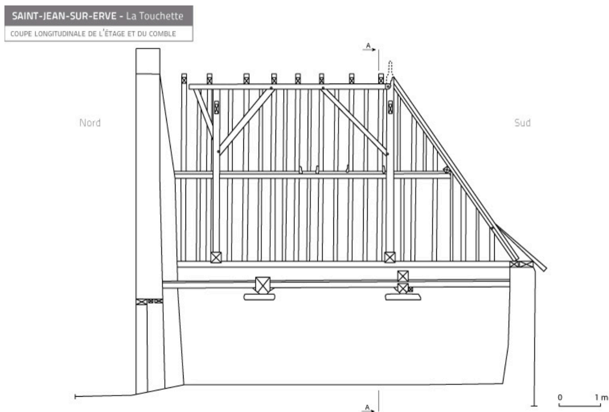
Coupe longitudinale de l'étage et du comble.
