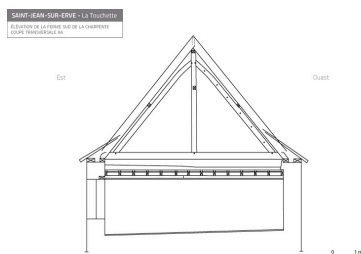
Charpente. Coupe transversale de la ferme sud. Dess. Laurent Cohin IVR52_20105300422NUDA
