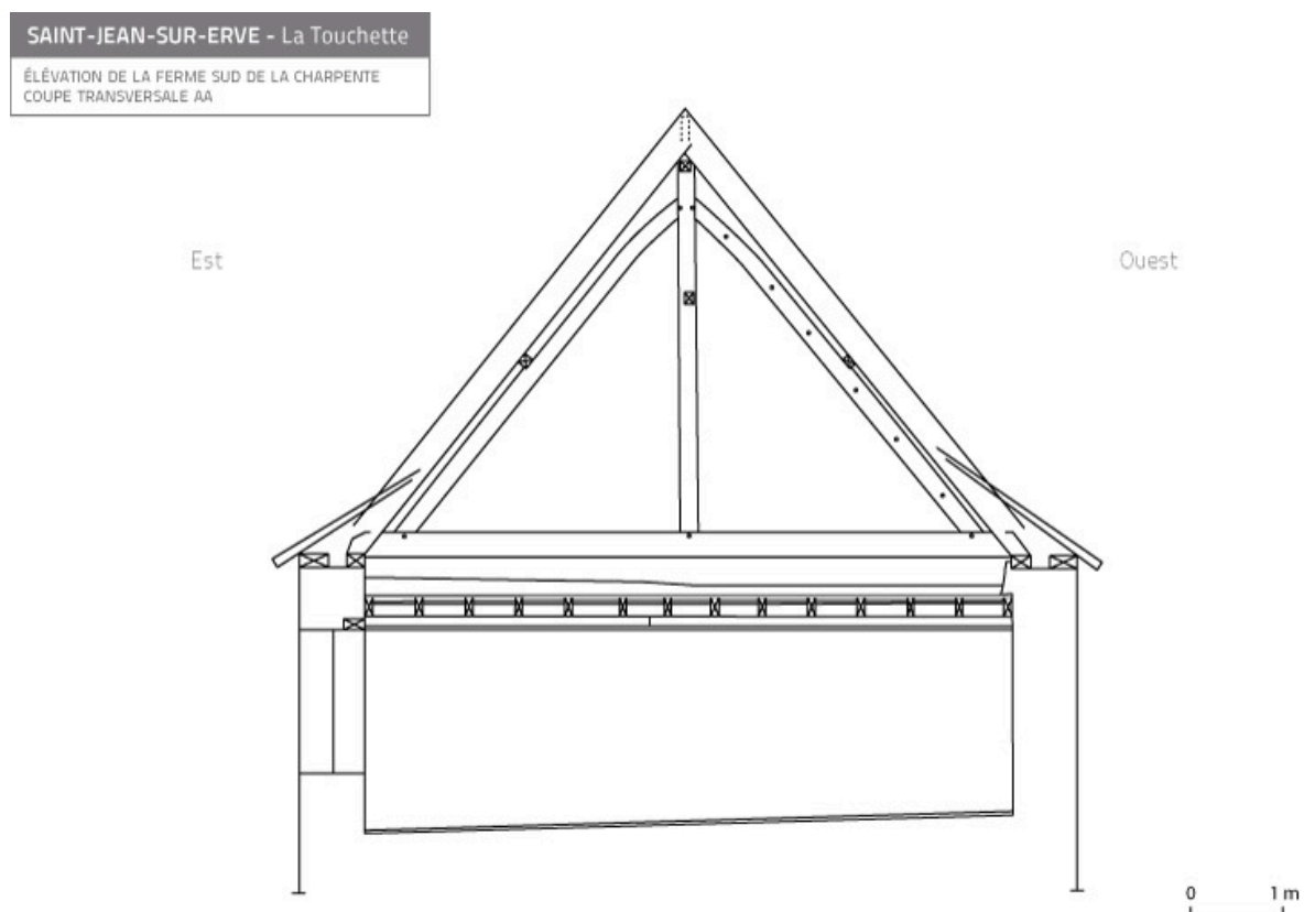
Charpente. Coupe transversale de la ferme sud.
