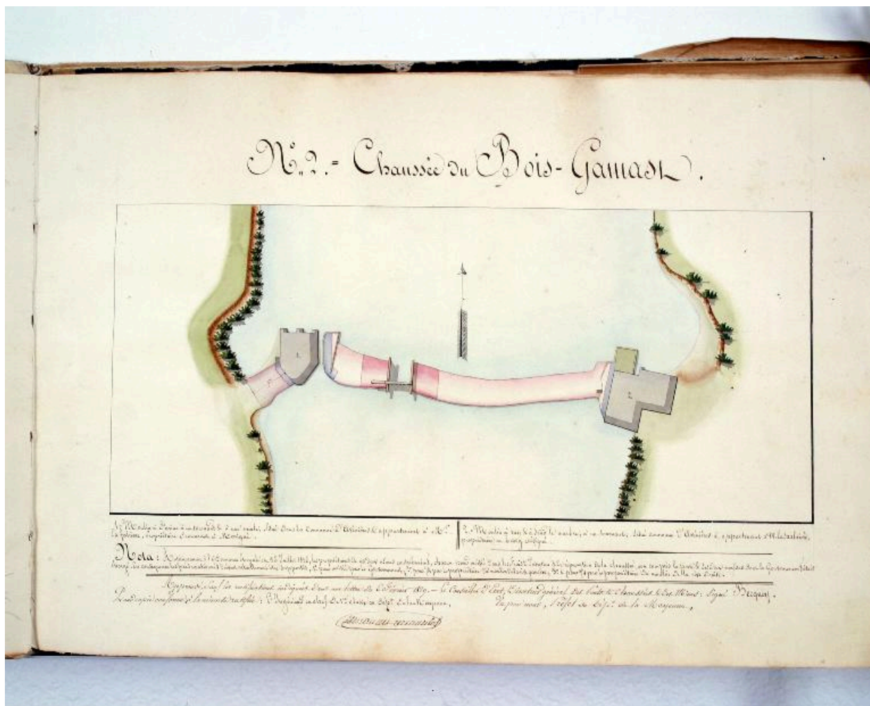
Planche n° 2 du recueil des plans des barrages de la partie navigable de la Mayenne. Plan d'ensemble du site du Bois-Gamats avant la canalisation de la rivière : barrage, porte marinière, moulin à farine du Bois-Gamats, moulin à tan du Gravier (supprimés).
