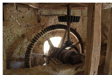
L'usine du moulin, r-d-c : détail d'un ancien mécanisme. Phot. Jean-Baptiste Darrasse IVR52_20107201357NUCA
