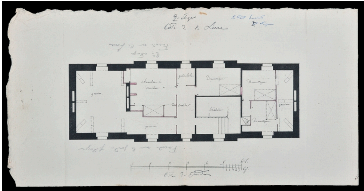
Plan de l'étage de comble. Vers 1808. (Archives départementales de Maine-et-Loire, 103 J 33/15).
