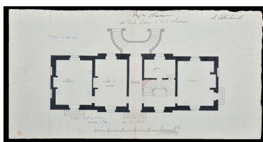
Plan du rez-de-chaussée surélevé. Vers 1808. (Archives départementales de Maine-et-Loire, 103 J 33/15). Repro. Bruno Rousseau IVR52_20164900105NUCA
