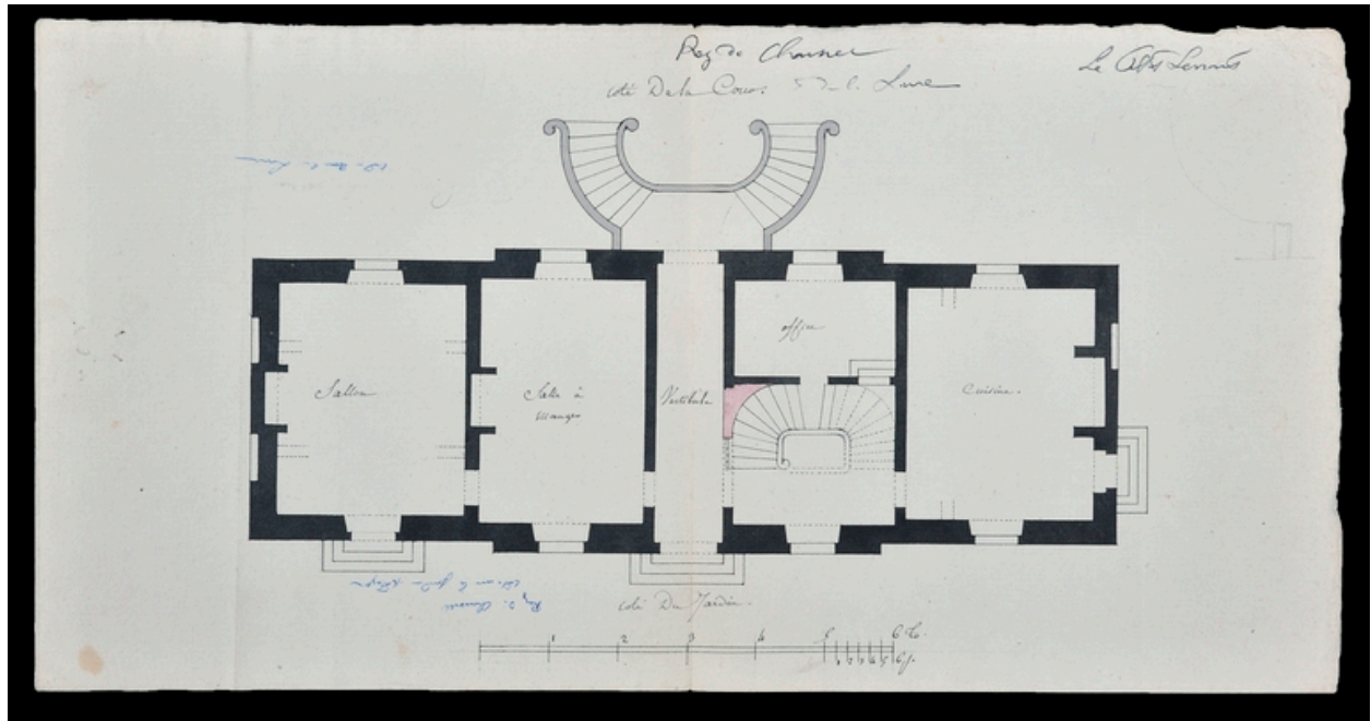
Plan du rez-de-chaussée surélevé. Vers 1808. (Archives départementales de Maine-et-Loire, 103 J 33/15).
