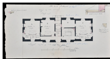
Plan du 1er étage. Vers 1808. (Archives départementales de Maine-et-Loire, 103 J 33/15). Repro. Bruno Rousseau IVR52_20164900106NUCA
