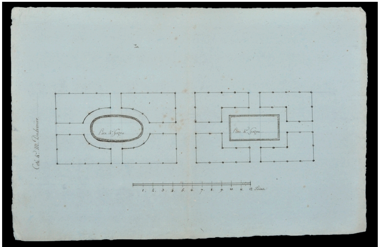
Plan de la première terrasse. Vers 1808. (Archives départementales de Maine-et-Loire, 103 J 33/15).
